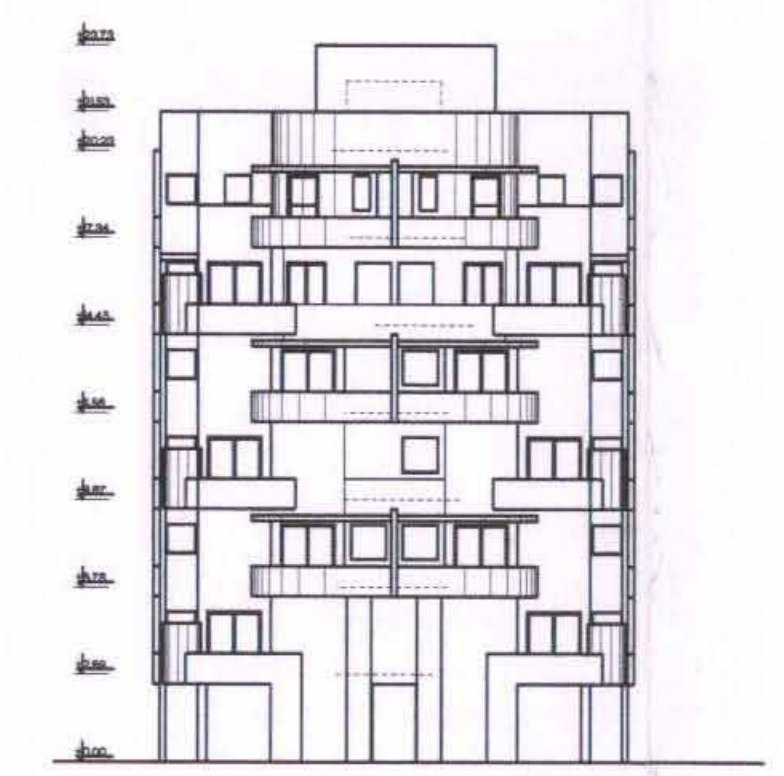
חזית מזרחית 1:250
