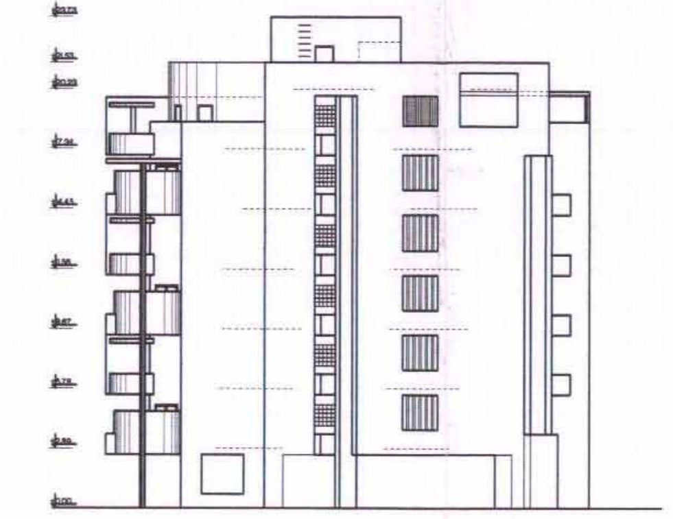
חזית צפונית 1:250
