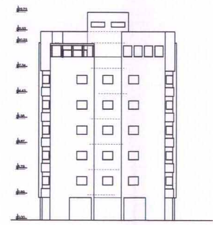
חזית מערבית 1:250
