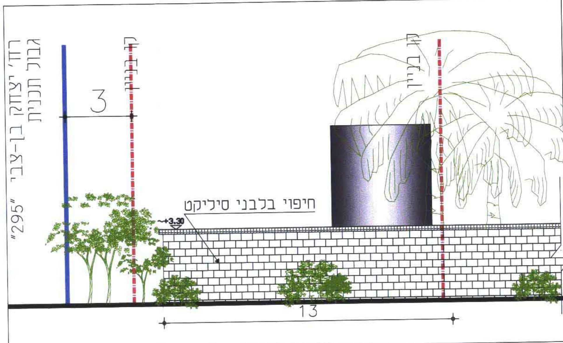
חזית מוצעת וחזית קיימת בתוספת כרכוב קנ"מ 1:100
