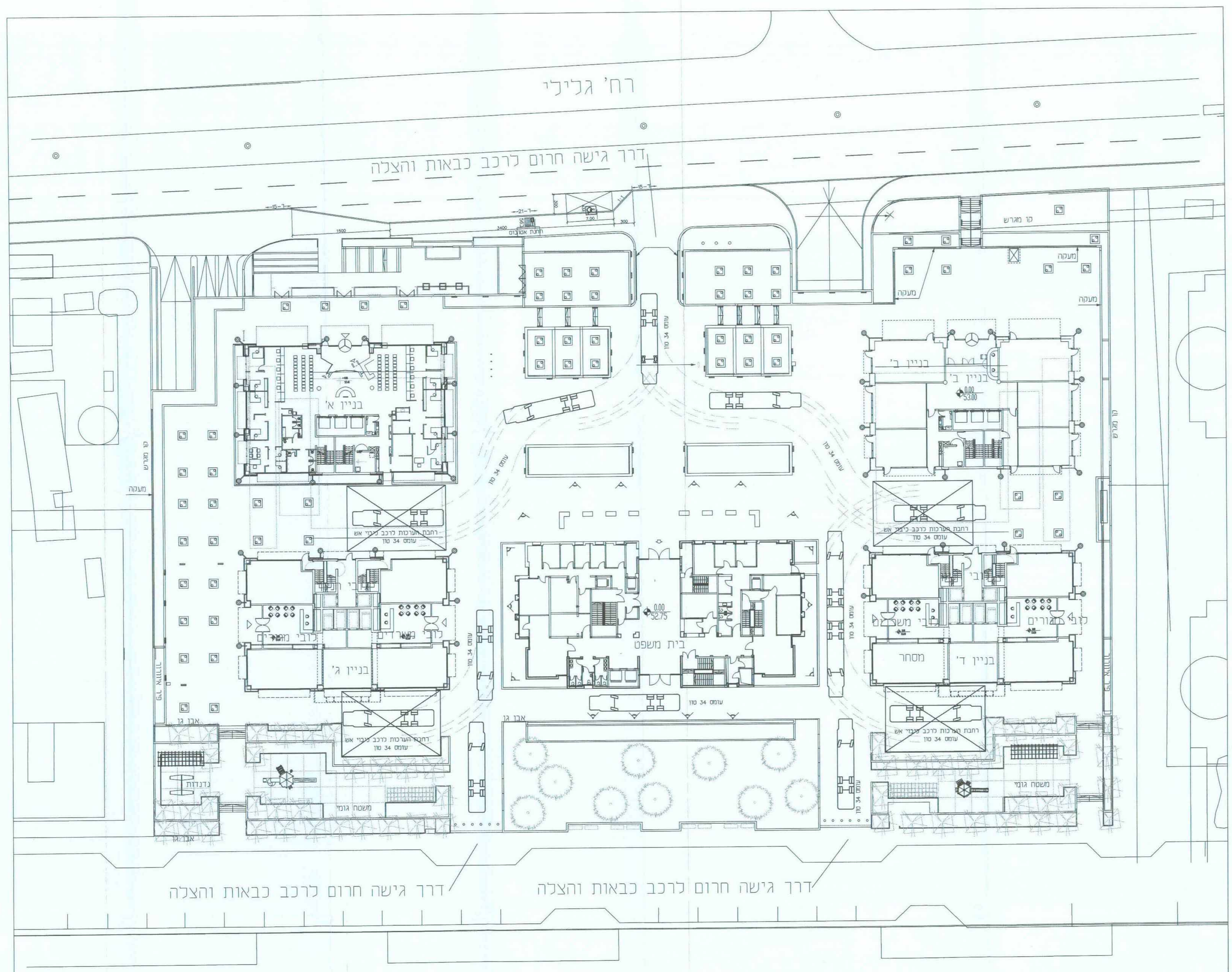
קומת קרקע 1 : 250 קני"מ
