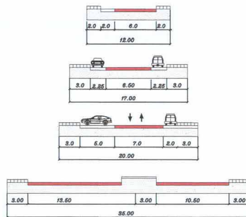
חיתוכים טיפוסיים
