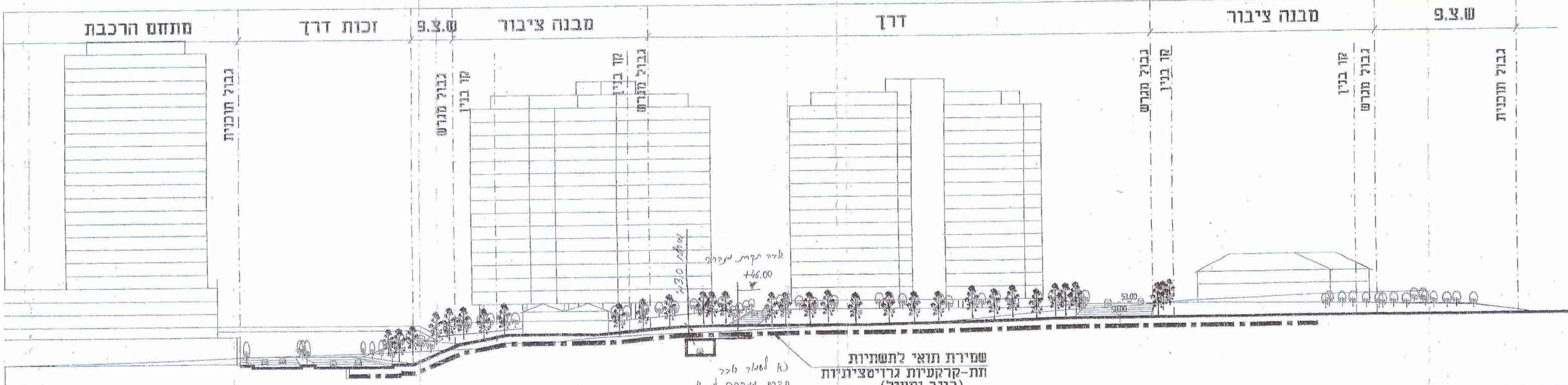
חתך B-B 1:625
