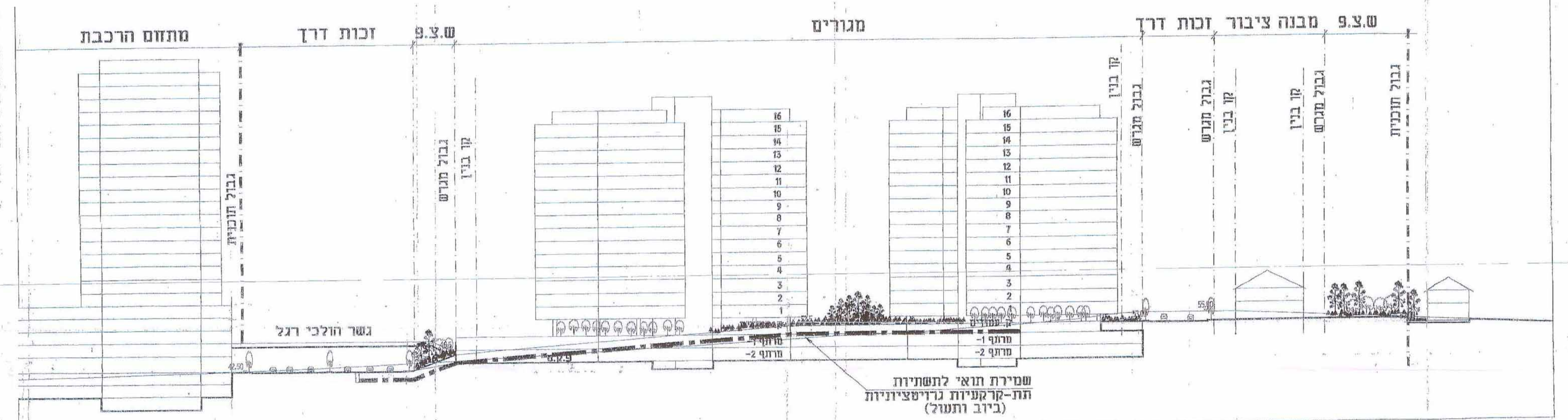
חתך A-A 1:625
