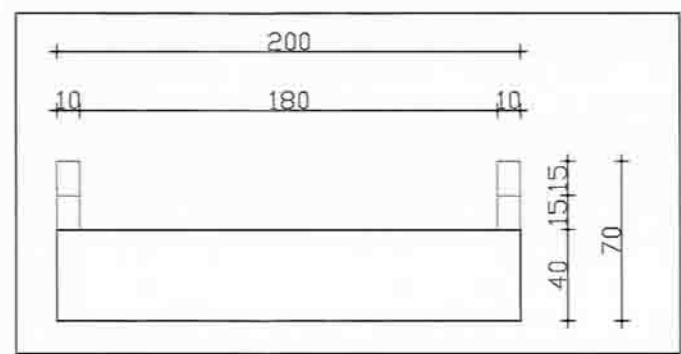
חזית צדדית
