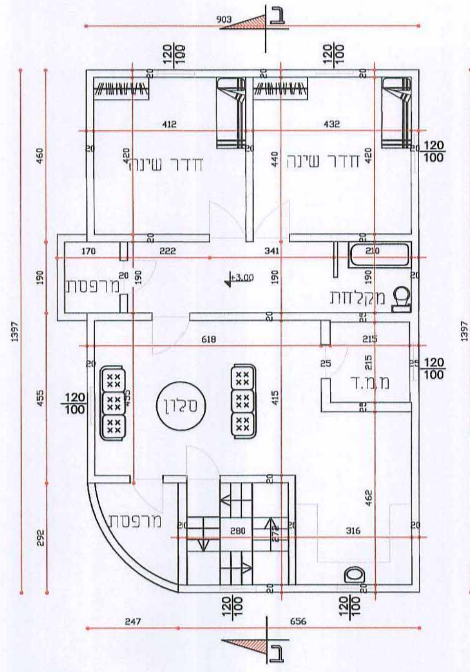
תוכנית קומה א' קנ"מ 1:100
