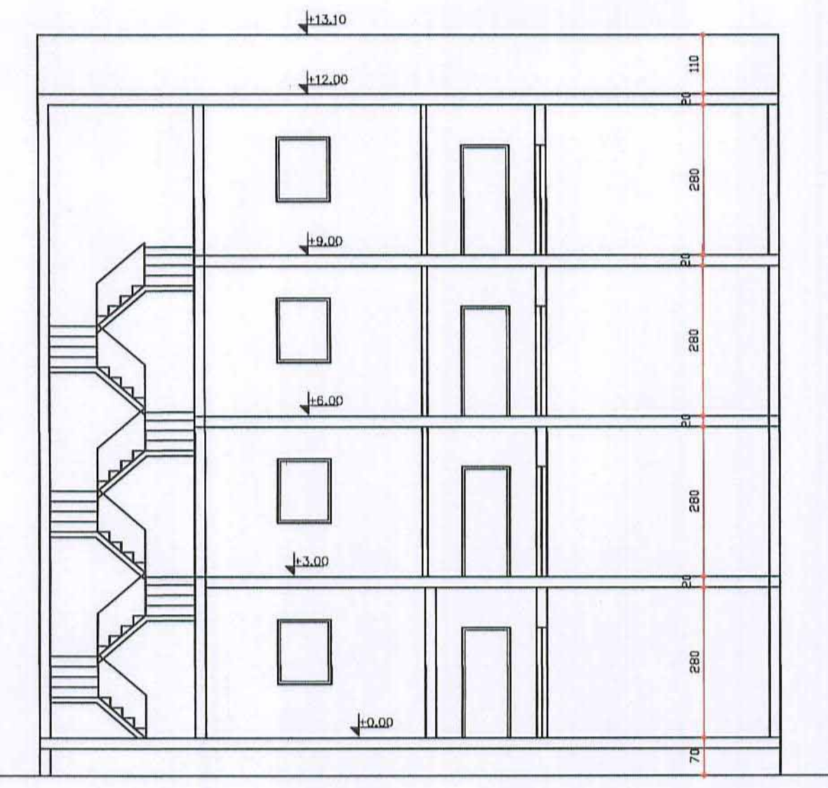
חתך ב-ב קנ"מ 1:100
