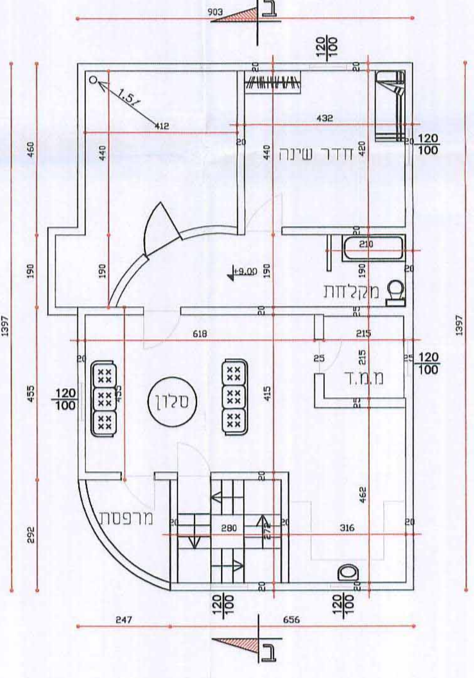
תוכנית קומה ג' קנ"מ 1:100
