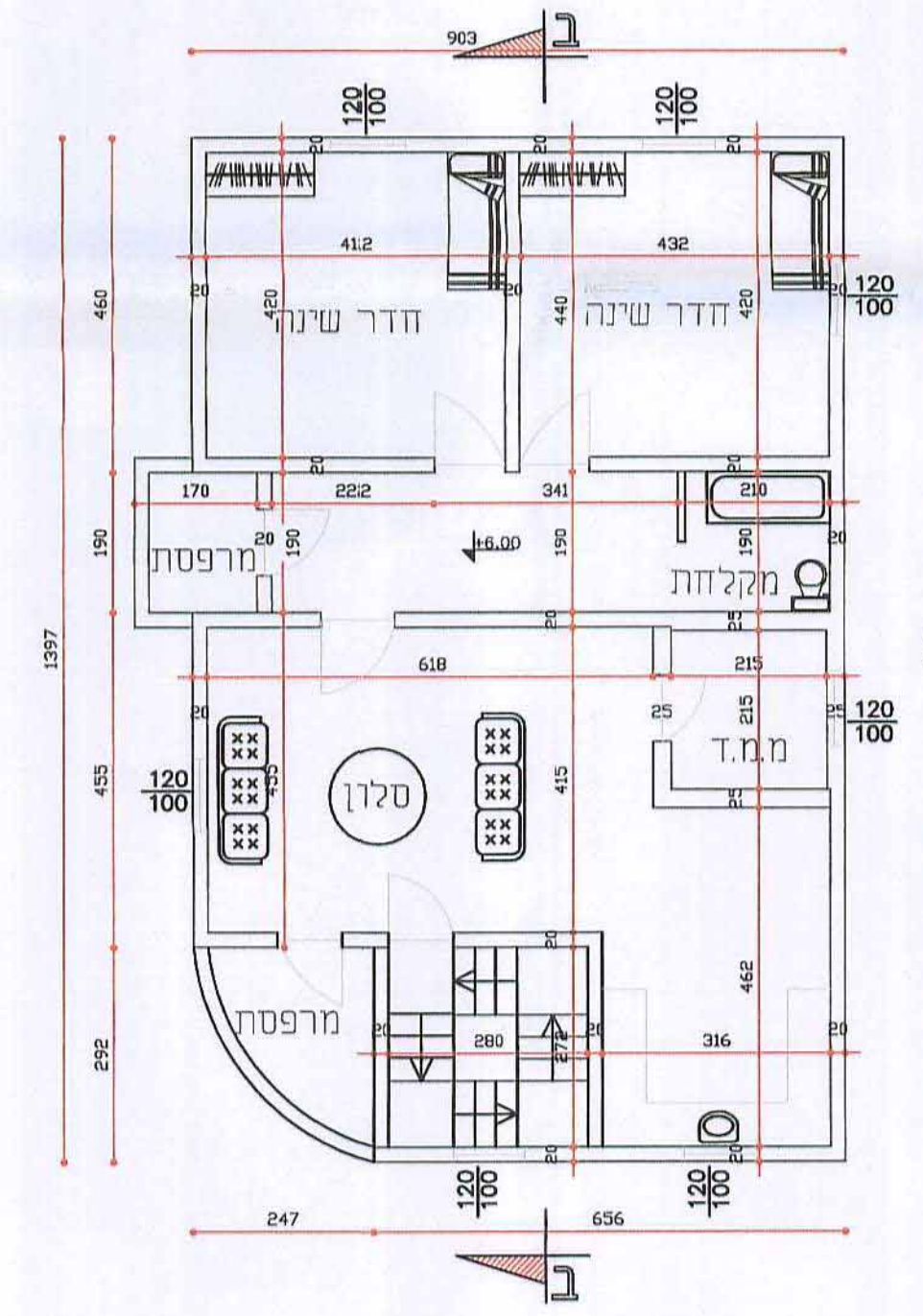
תוכנית קומה ב' קנ"מ 1:100
