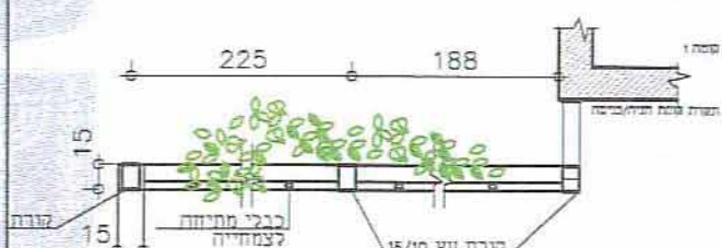
פרט פרגולה קנ"מ 1:50
