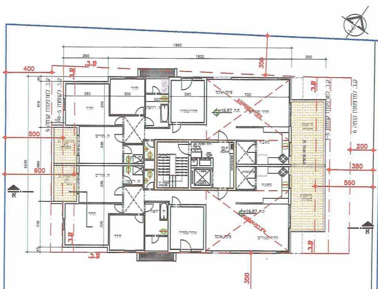
תוכנית קומה חמישית קנ"מ 1:200
