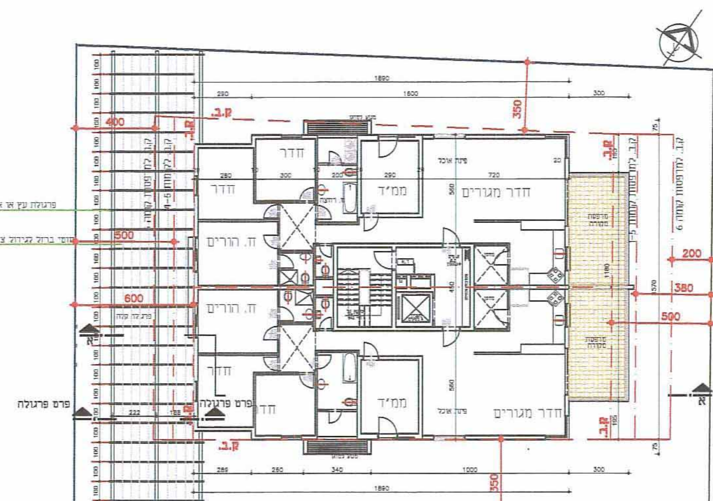
תוכנית קומה שיפוטית ראשונה- שלישית קנ"מ 1:200
