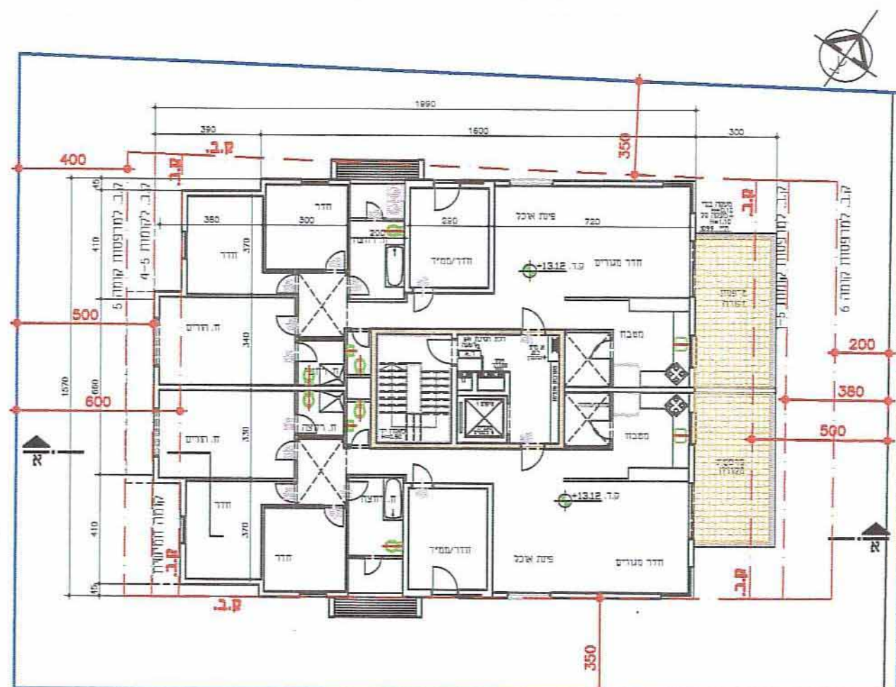
תוכנית קומה רביעית קנ"מ 1:200
