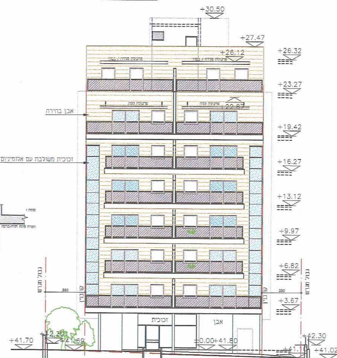
חזית מזרחית (ראשית) קנ"מ 1:200
