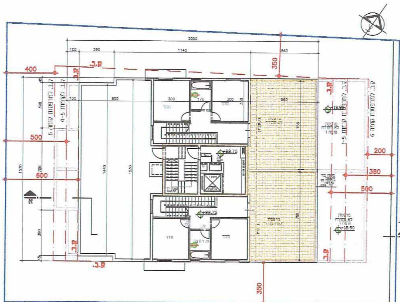
תוכנית חדרי גג קנ"מ 1:200
