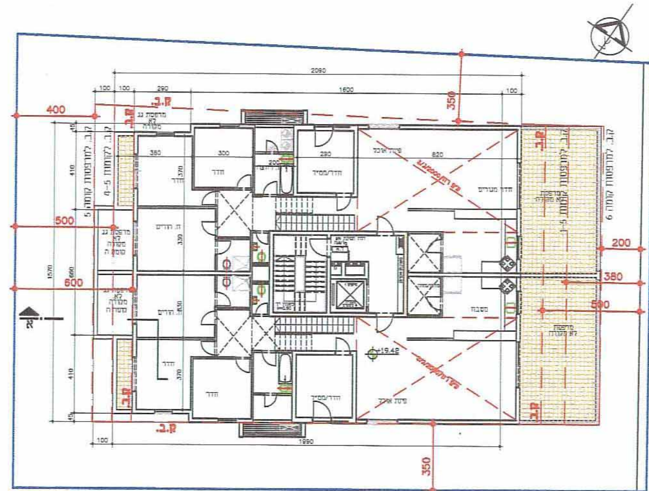
תוכנית קומה שיטית קנ"מ 1:200
