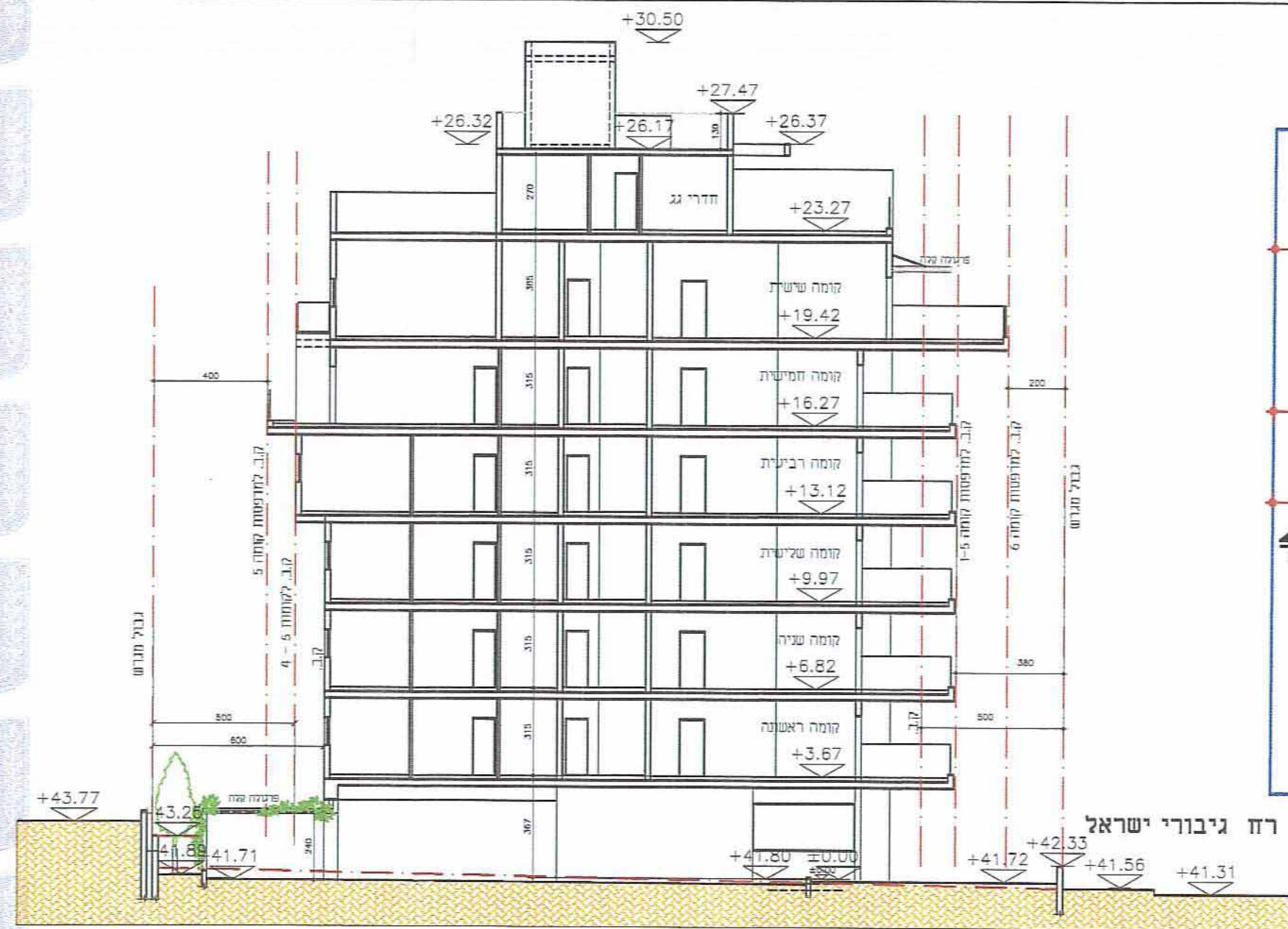
חיתוך א-א
