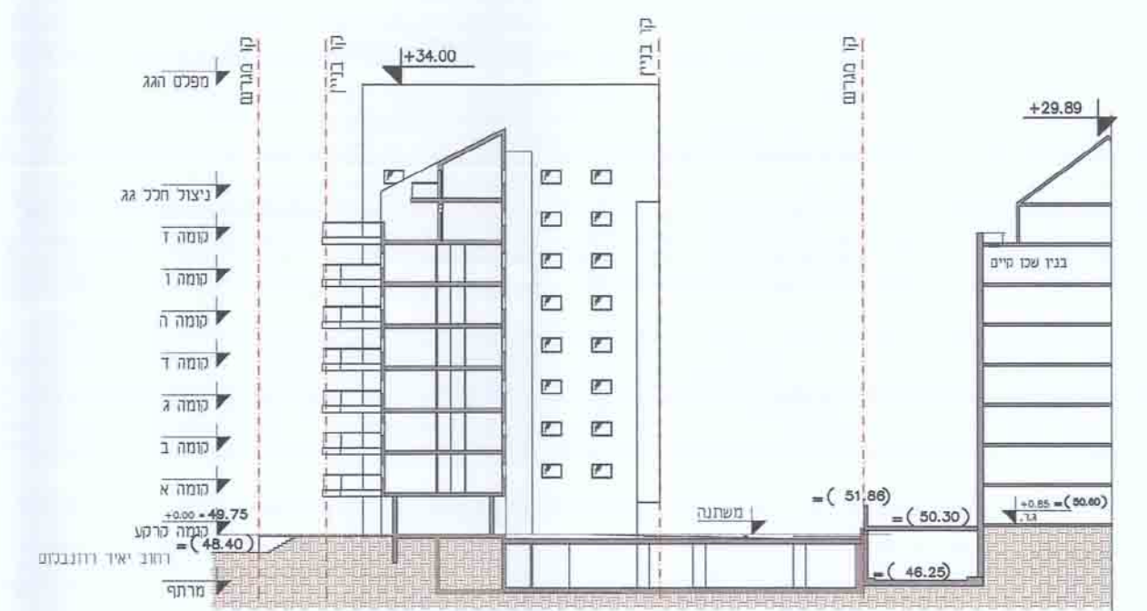
חזית עקרוני 1-1 1:250
