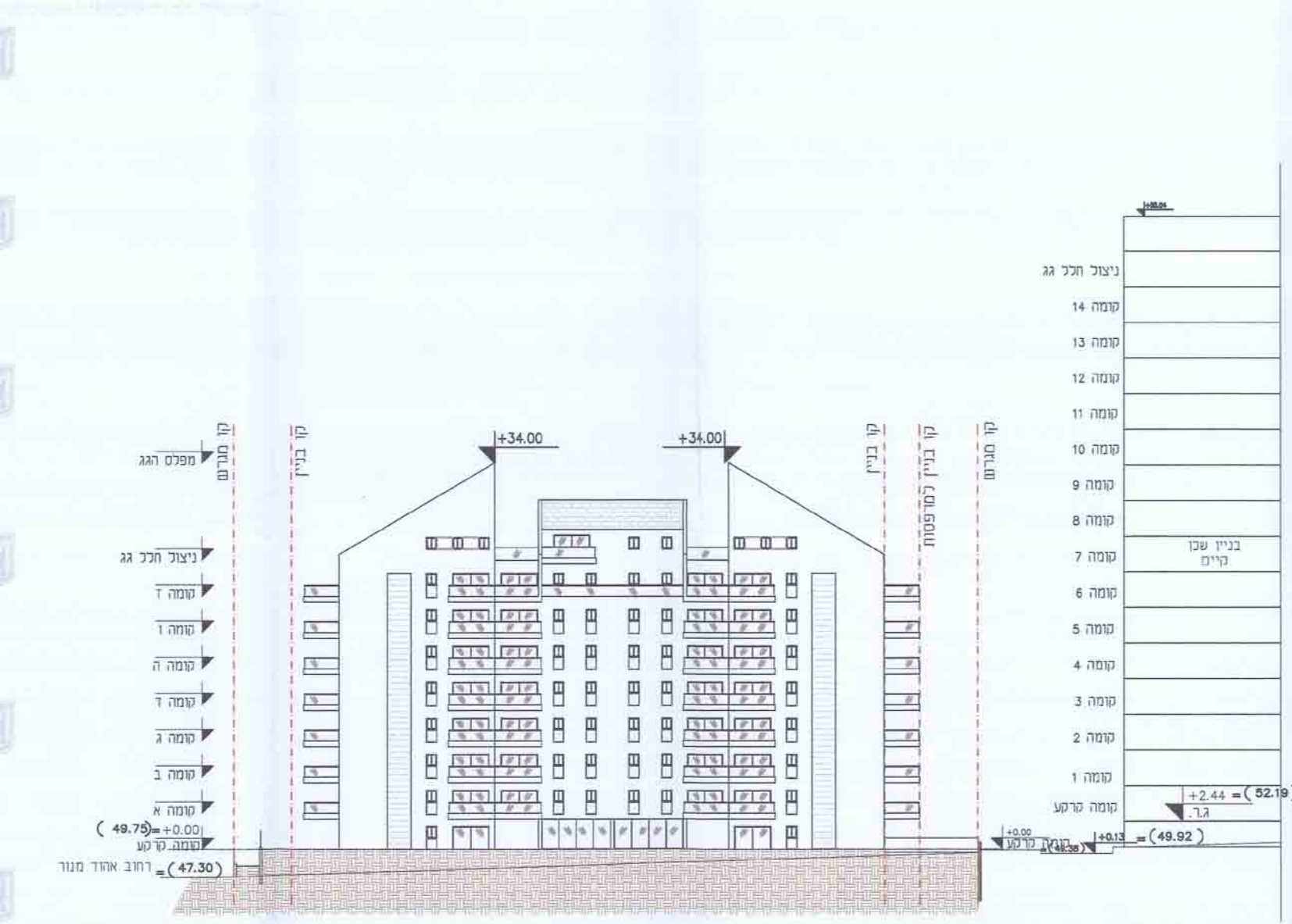
חזית לרחוב יאיר רוזנבלום 1:250
