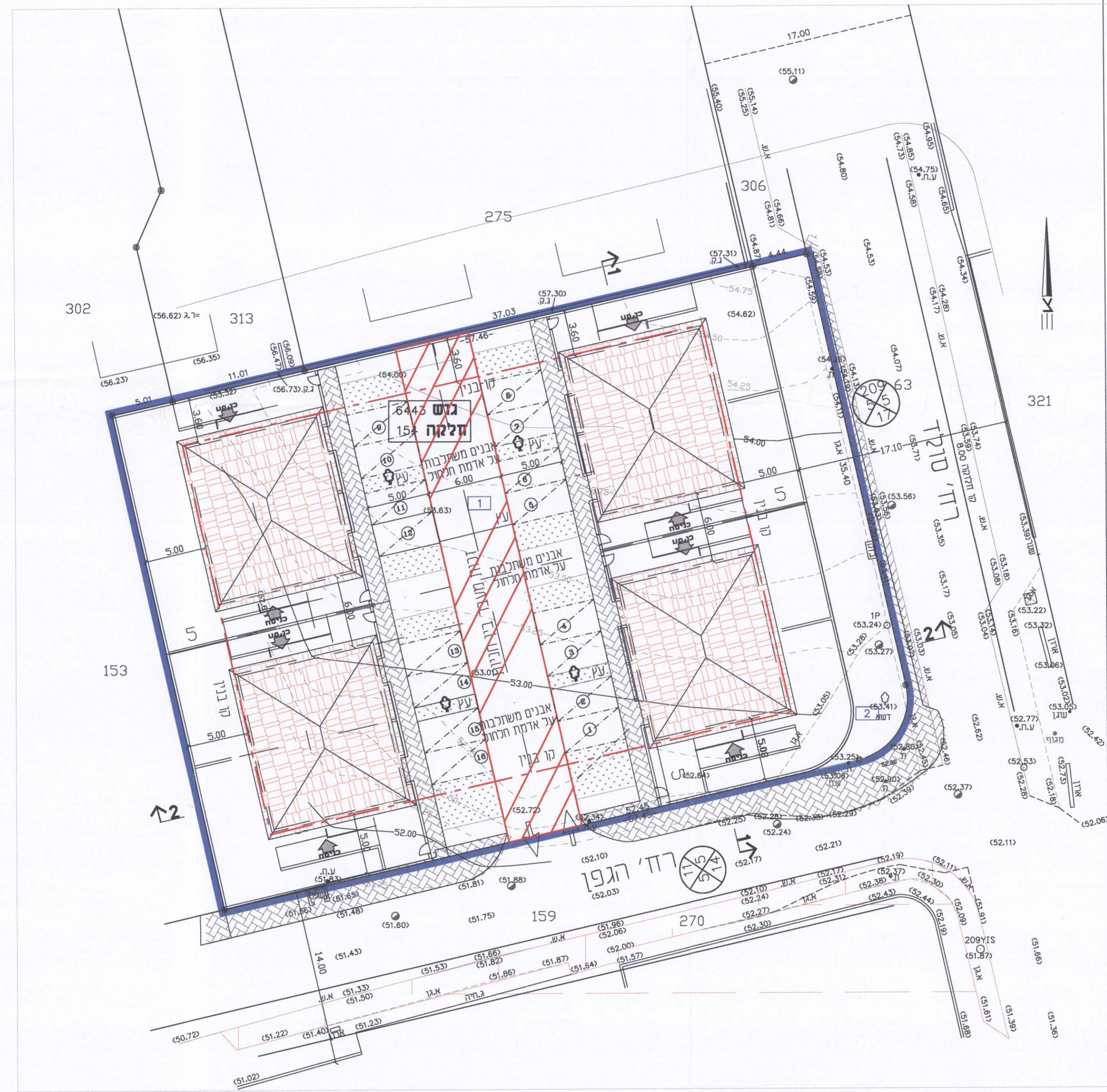
תכנית בינוי עקרונית מנחה נספח תנועה וחניה-מחייב לכניסה לזכות מעבר מרחי' הגפן 1: 250
