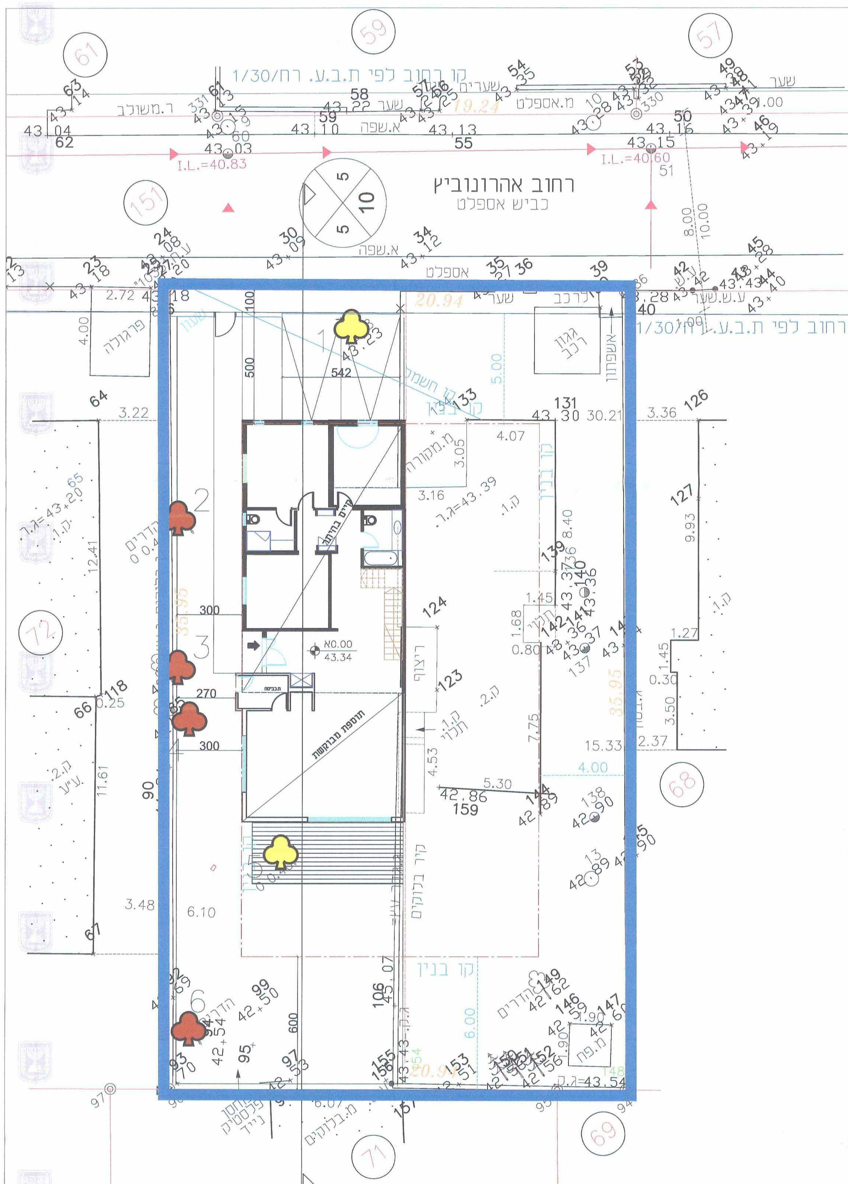
בית משפחת צעדי - תכנית קומת קרקע
