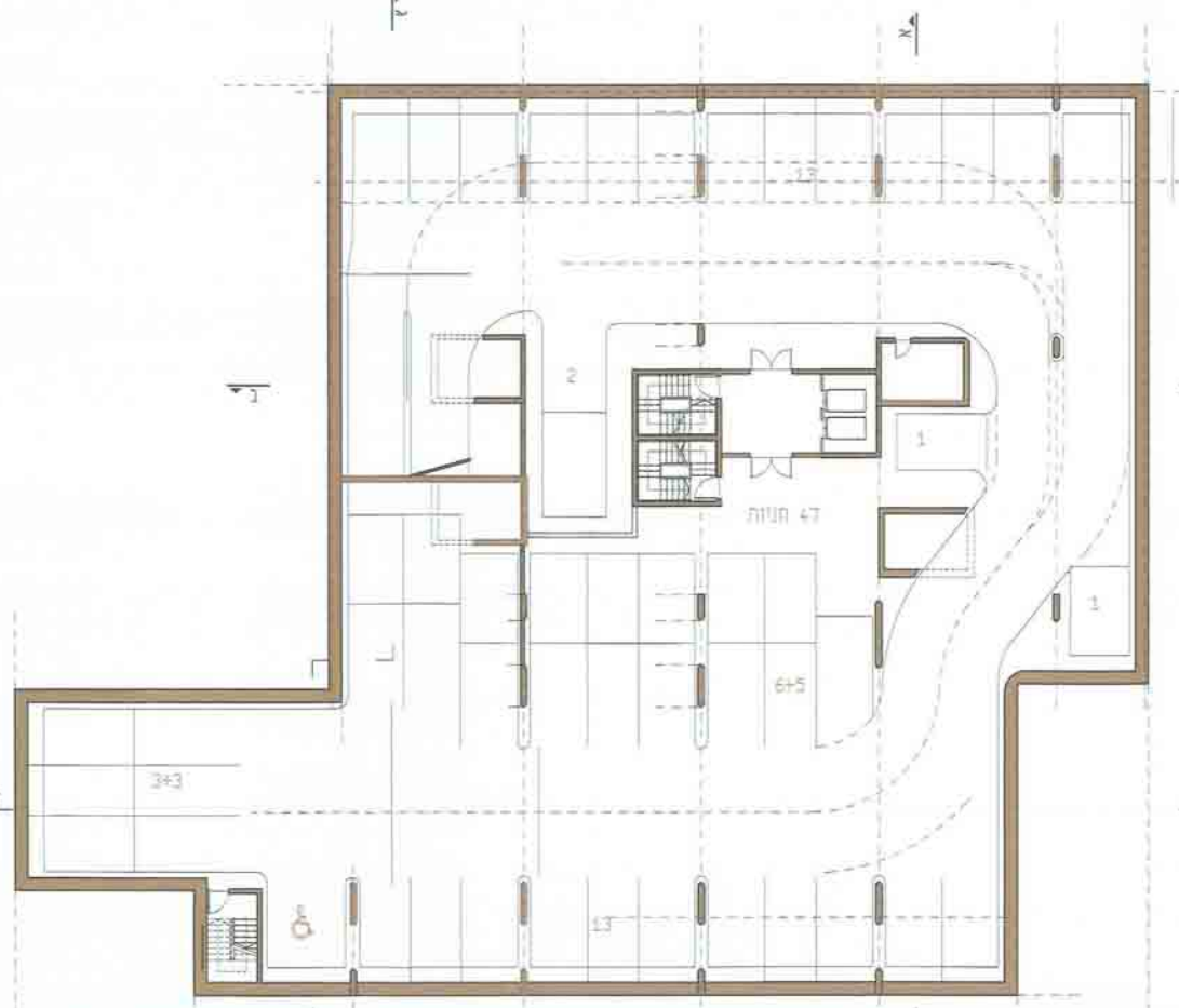
תכנית קומת מרתון 2 1-200
