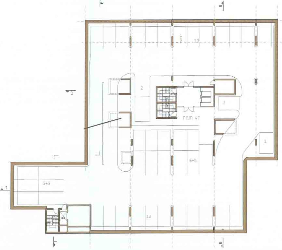
תכנית קומת מרתון 1 1-200
