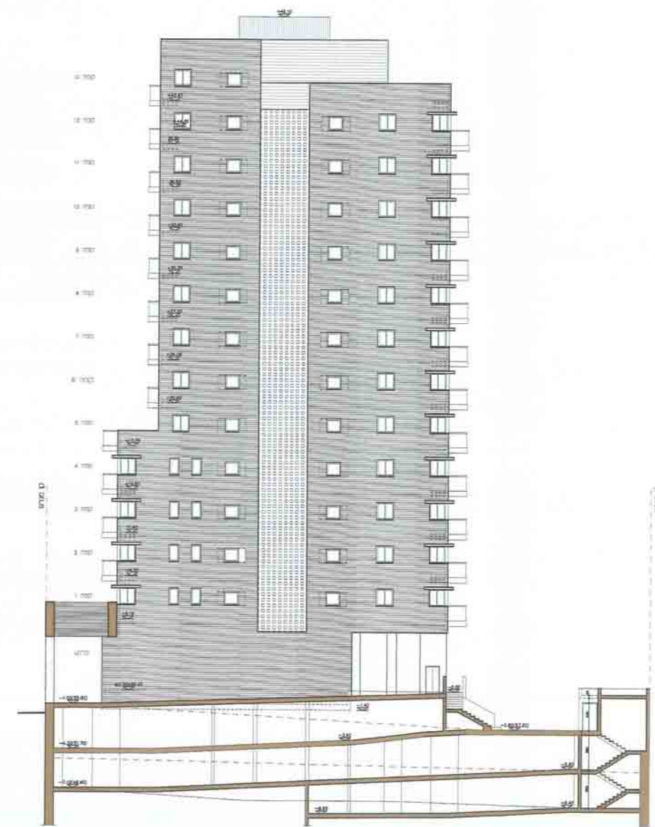
חזית צד מזרחית 1-200
