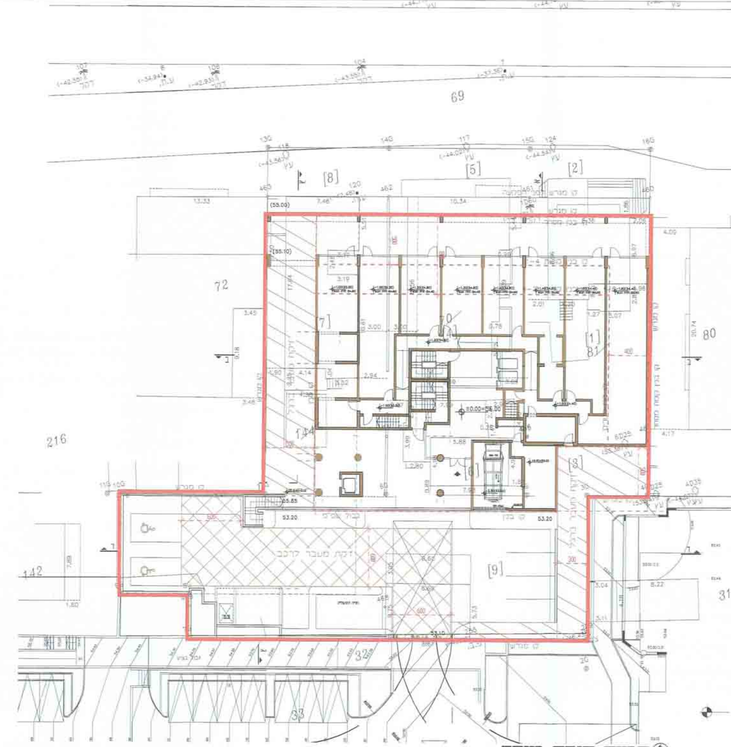
תכנית קומת כניסה 1-200
