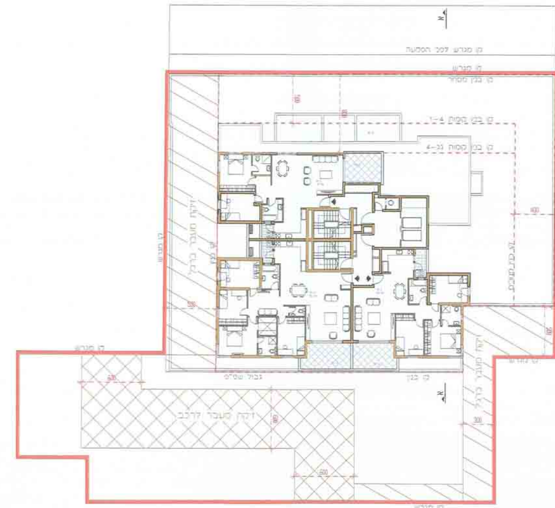
תכנית קומות טיפוסיות 5 - 12 1-200
