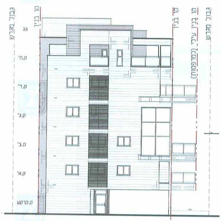
חזית דרום-מזרחית קני"מ 1:200
