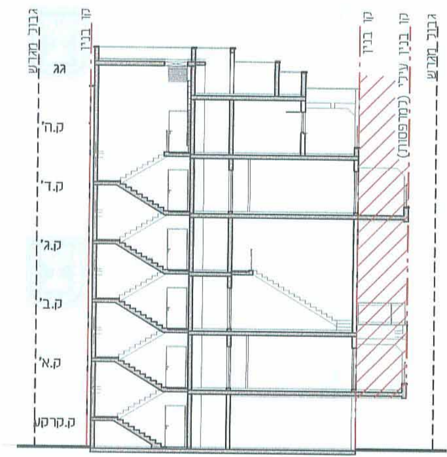
חיתך 2-2 (טיפוסי) קני"מ 1:200
