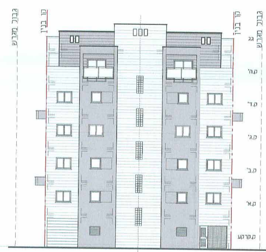
חזית דרום-מערבית קני"מ 1:200
