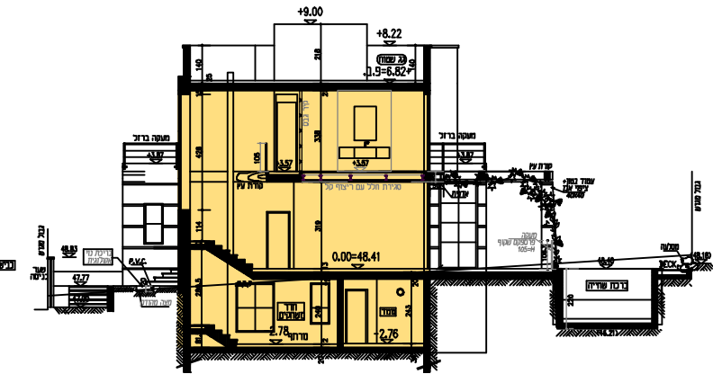
חתך א-א, ק.מ. 1:250
