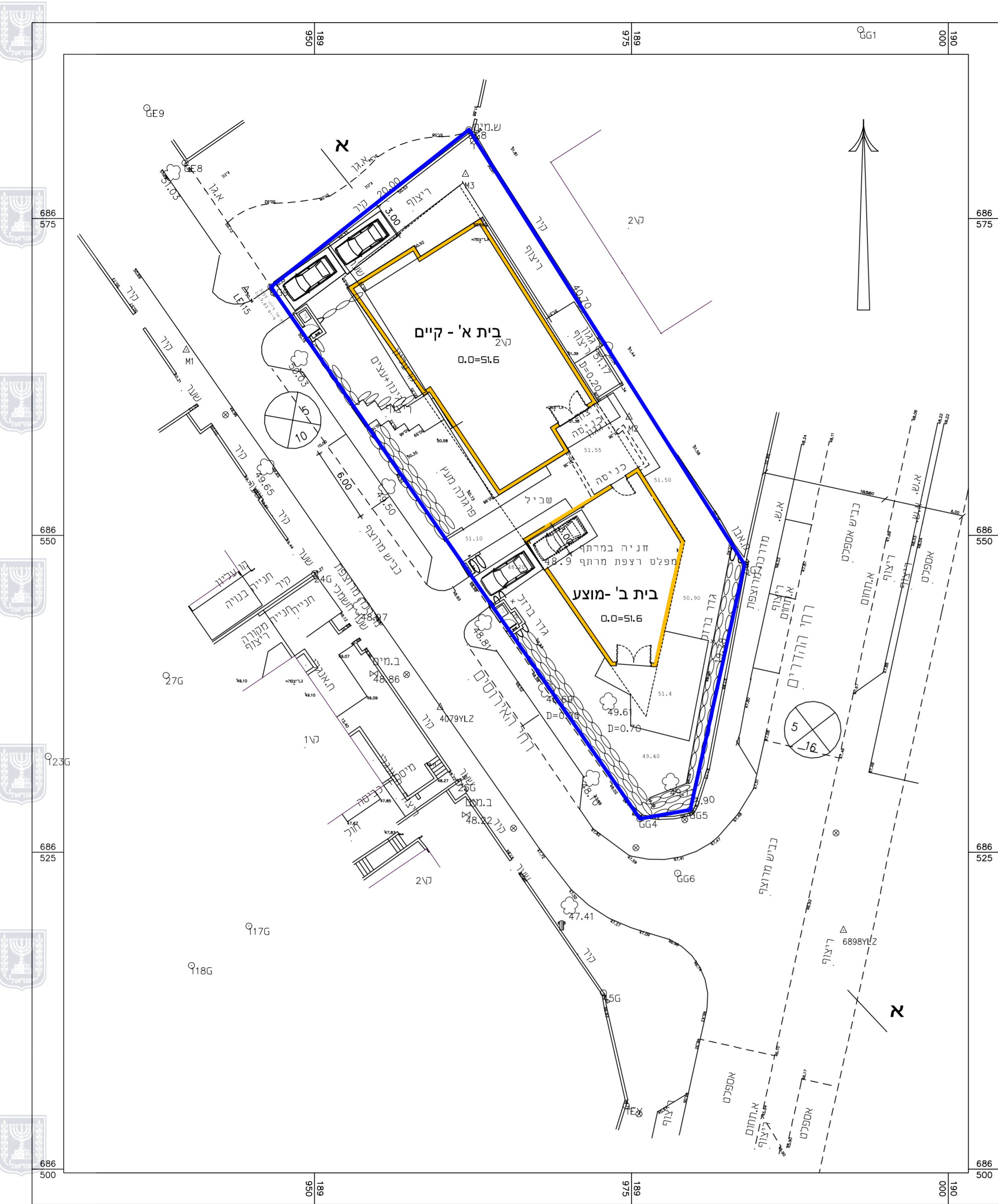
תשריט בינוי 1:250
