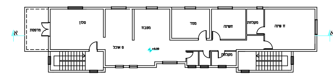
תוכנית קומה ב' קנ"מ 250:1
