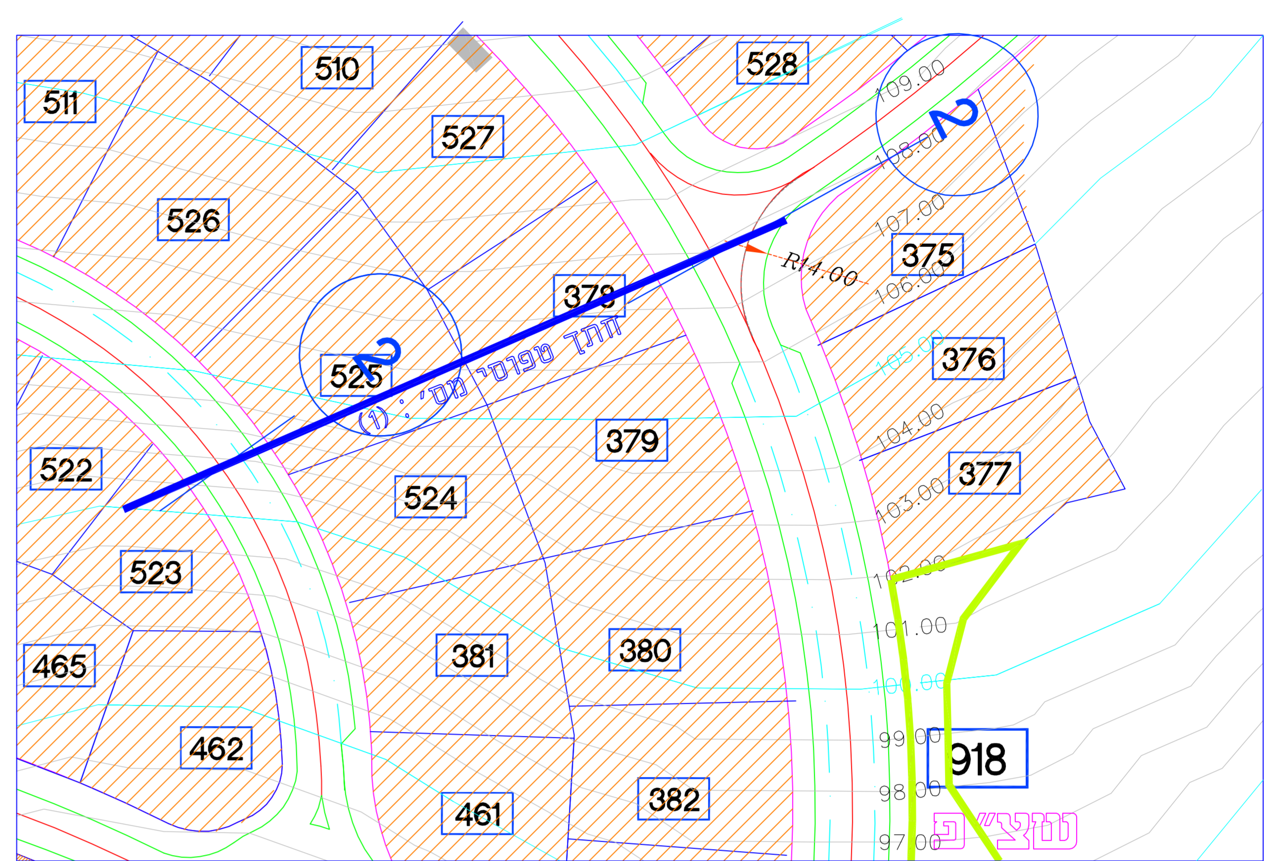
חתך טפוסי מס' (1)
