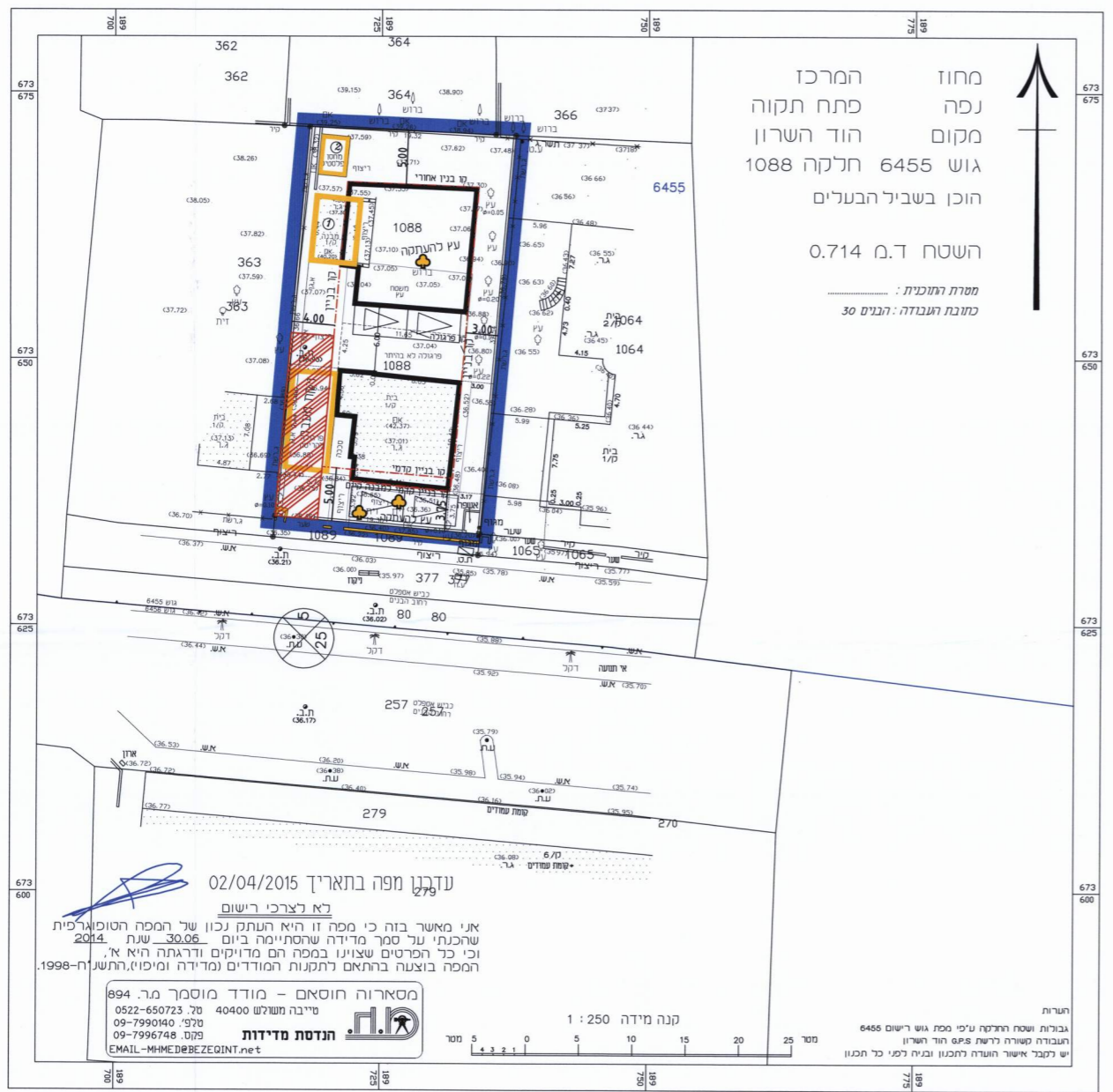
מצב מוצע קני"מ 1 : 250
