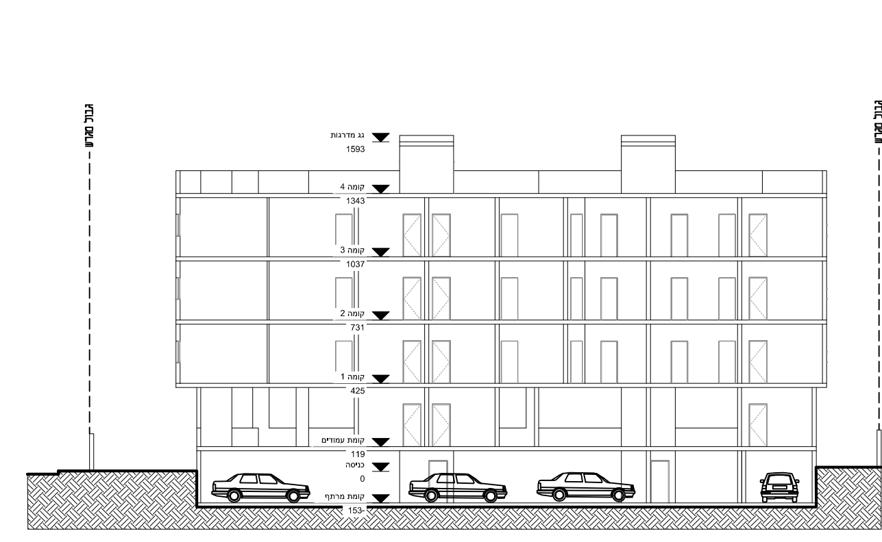
חתך ב-ב 1 : 250
