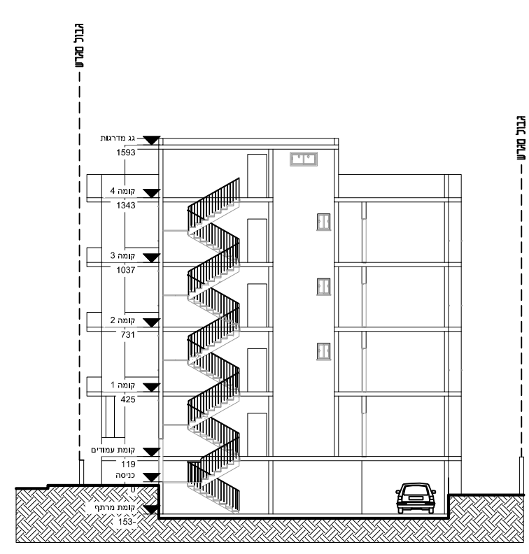
חתך א-א 1 : 250
