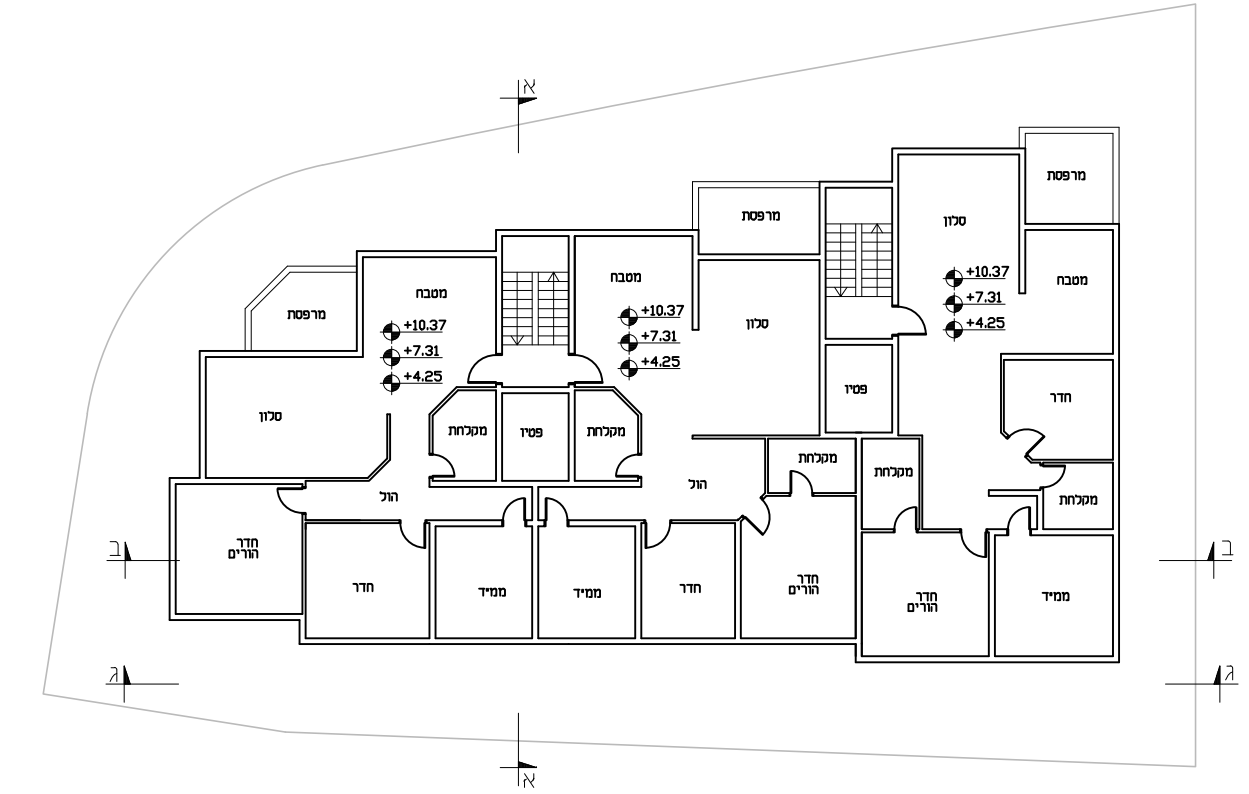
תכנית קומות 1-3 1 : 250
