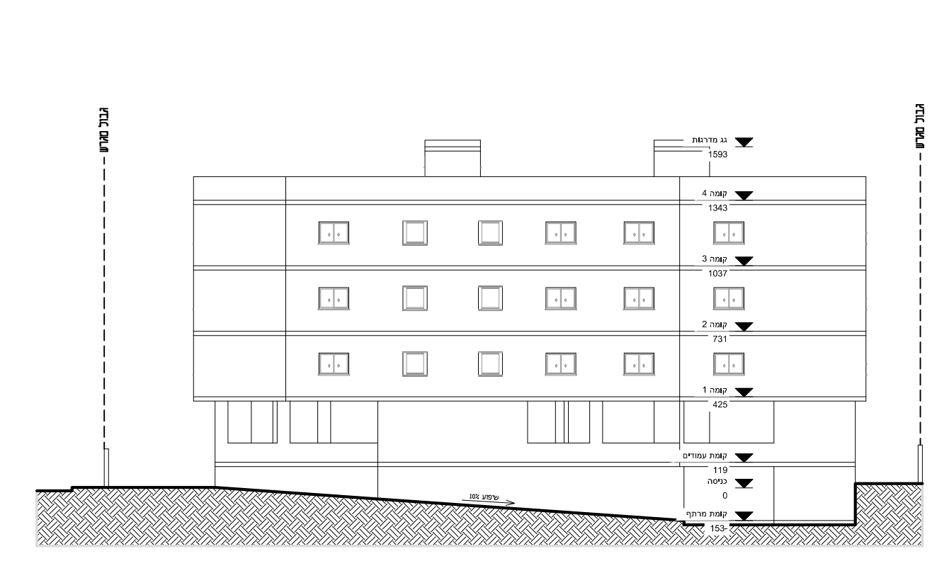
חתך ג-ג 1 : 250
