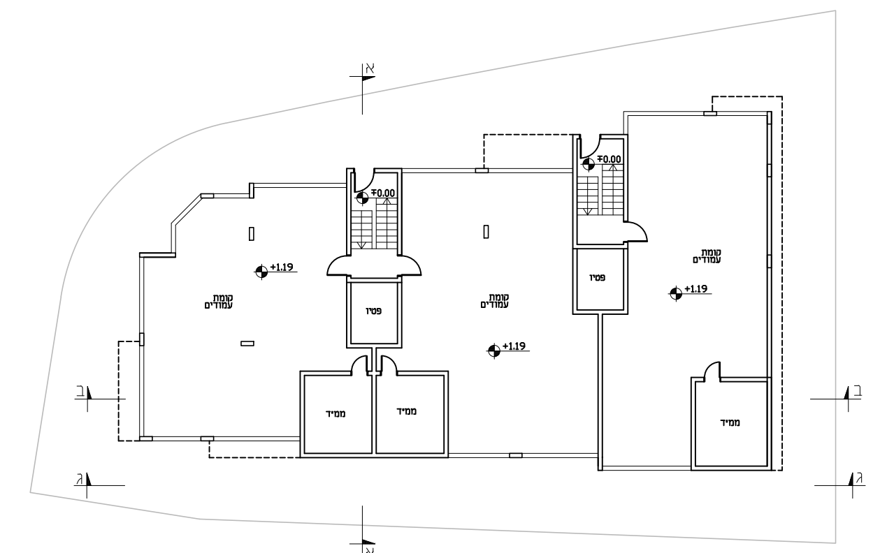
תכנית קומ' 1 : 250
