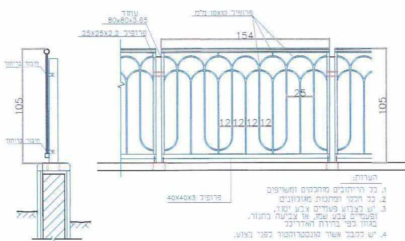
פרט גדר אופיינית קני"מ 1:20
