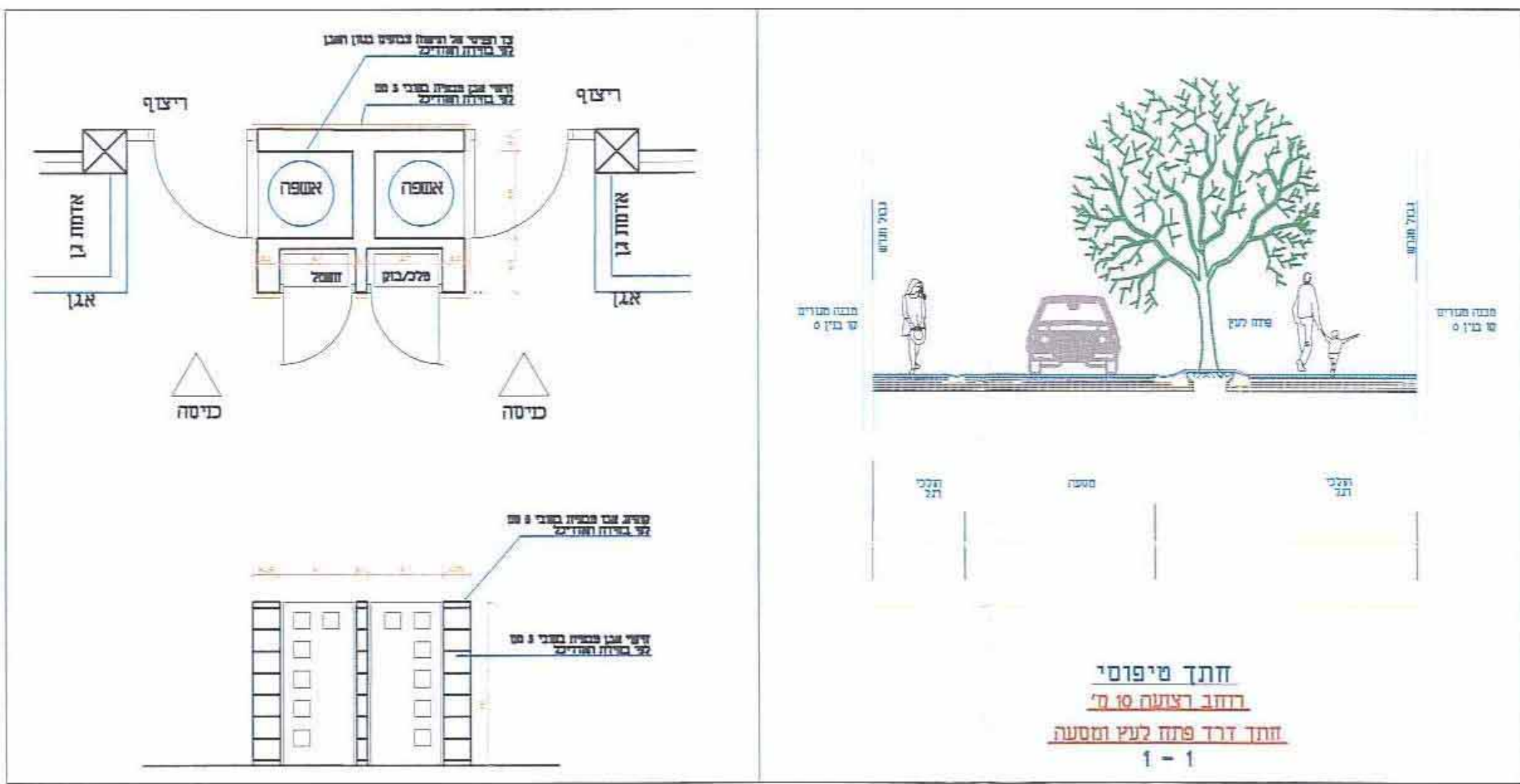
כניסה אופיינית קני"מ 1:50
