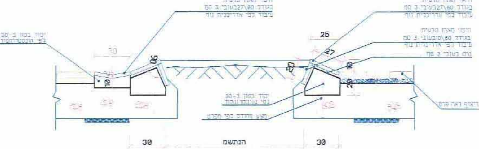
ציפוי קיר באבן טבעית
