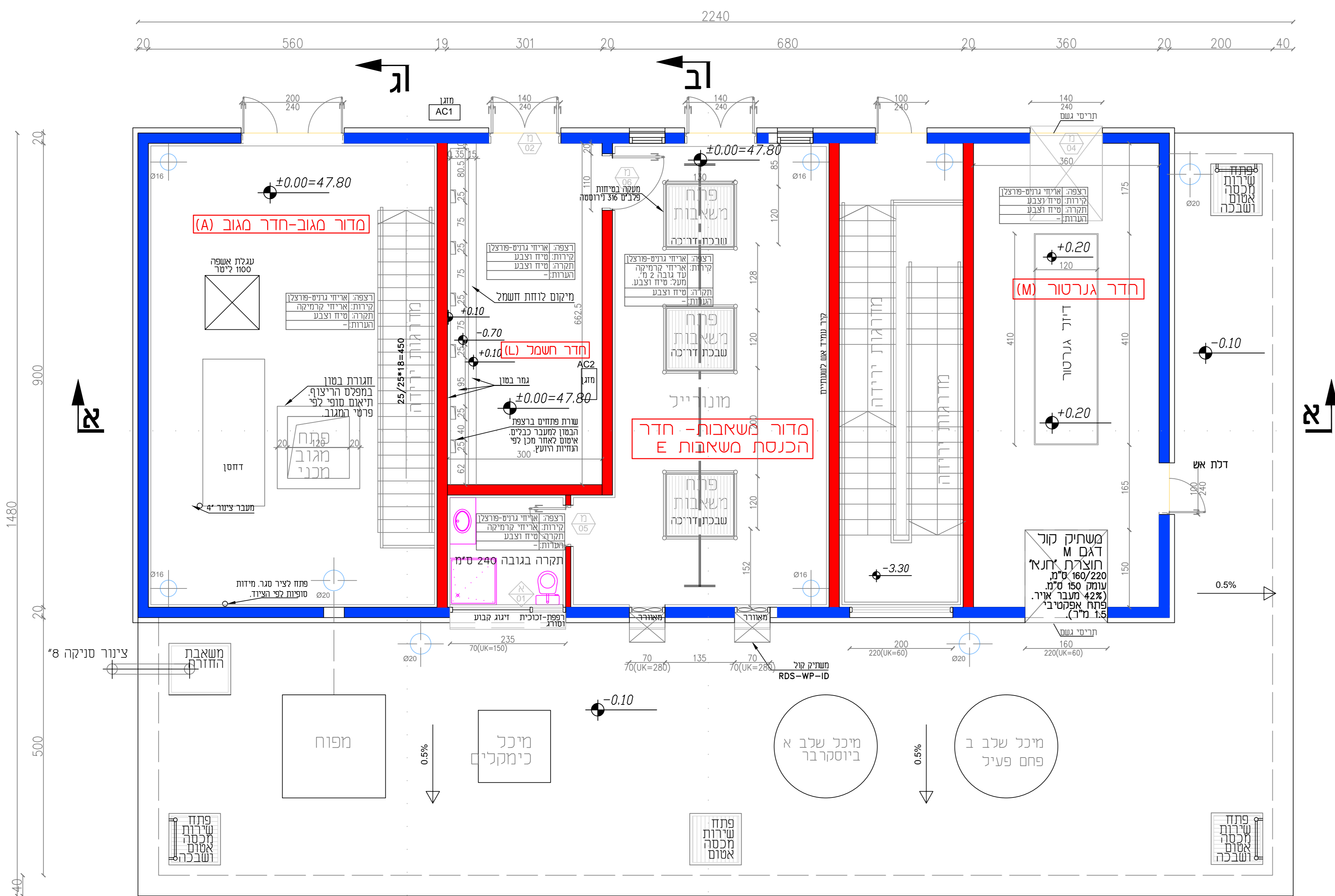
תכנית מפלס כניסה +0.00
