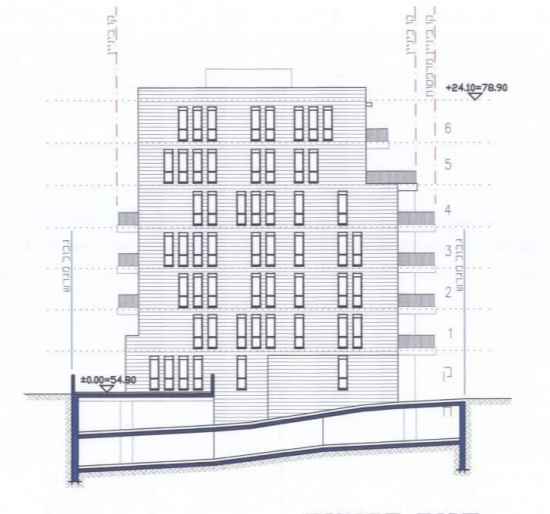
חזית דרומית
