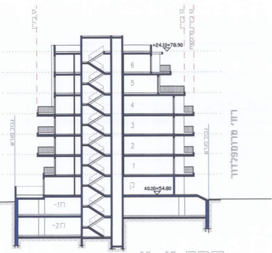
חתך א-א
