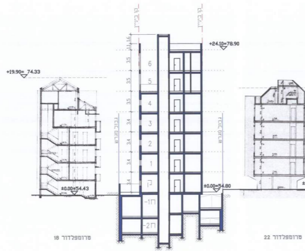
חתך ב-ב
