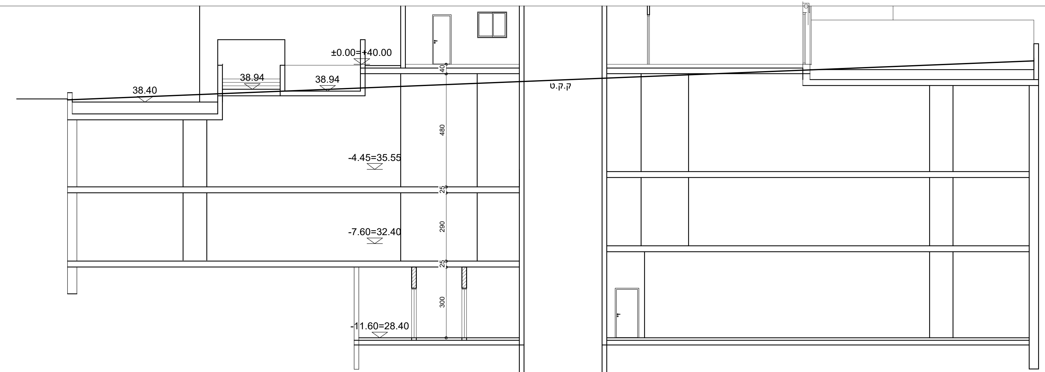
חתך 3-3 קנ"מ1:100
