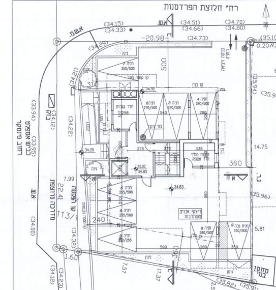
תוכנית קומות קרקע קני"ח 200 : 1
