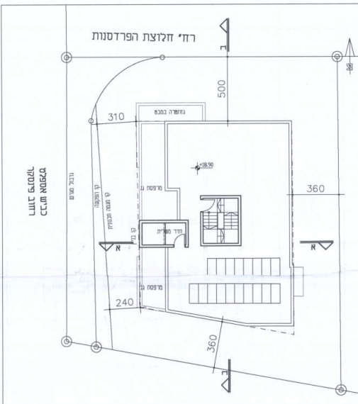
קומת גג עליזן קנ"מ 1 : 200
