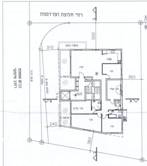
תוכנית קומת ג. ק"מ 1 : 200
