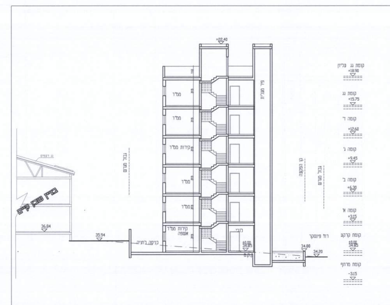
חתך א'-א' קנ"ם 1 : 200
