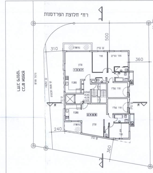
מכונת קומות א'-ד' 1:200 מ"מ
