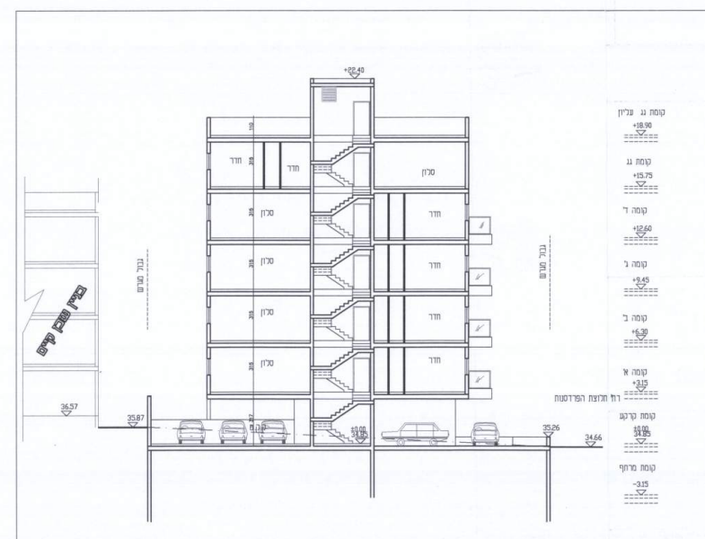
חתך ב'-ב' קני"ם 1 : 200
