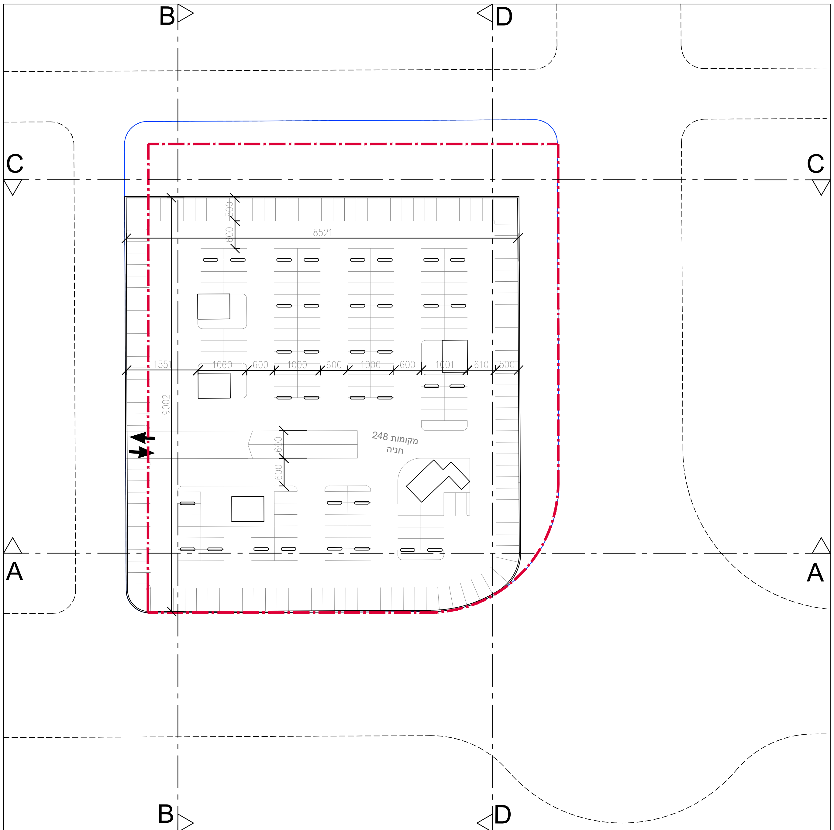
תכנית מרתפים
