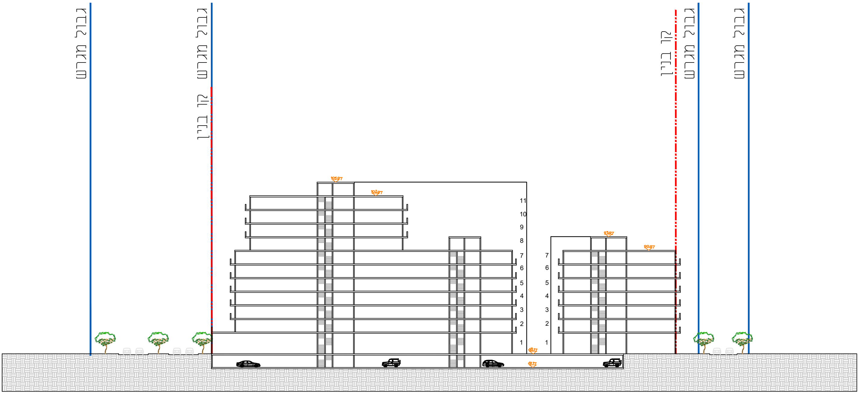
D-D חתך
