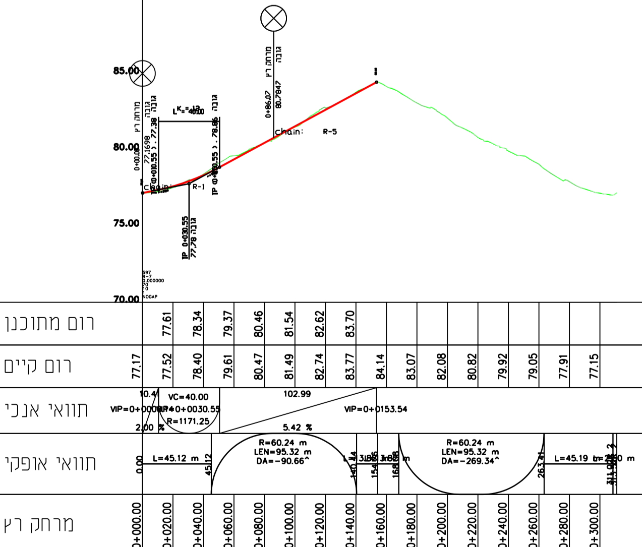
חתך לאורך דרך מסי' 07
