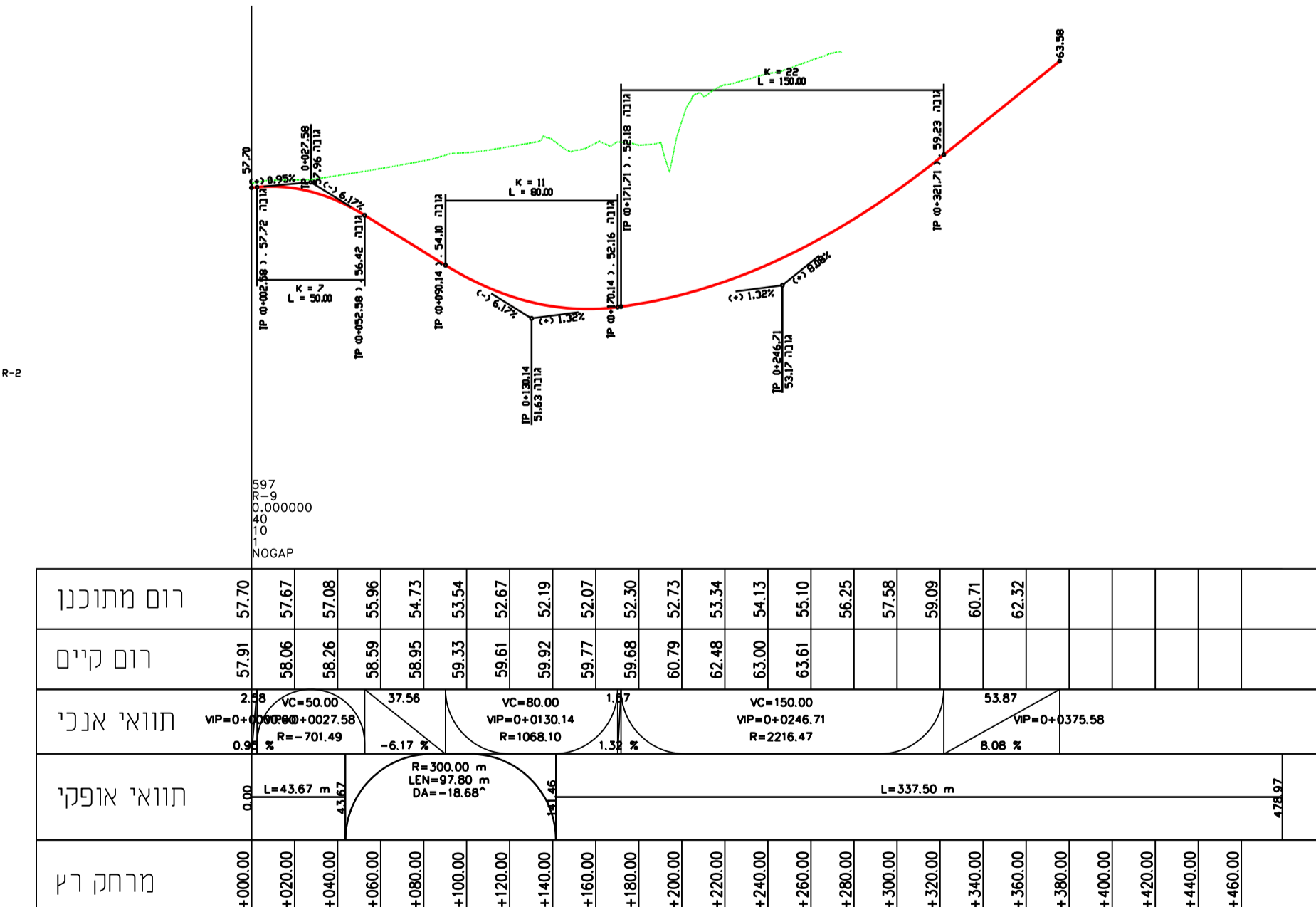
חתך לאורך דרך מסי' 09
