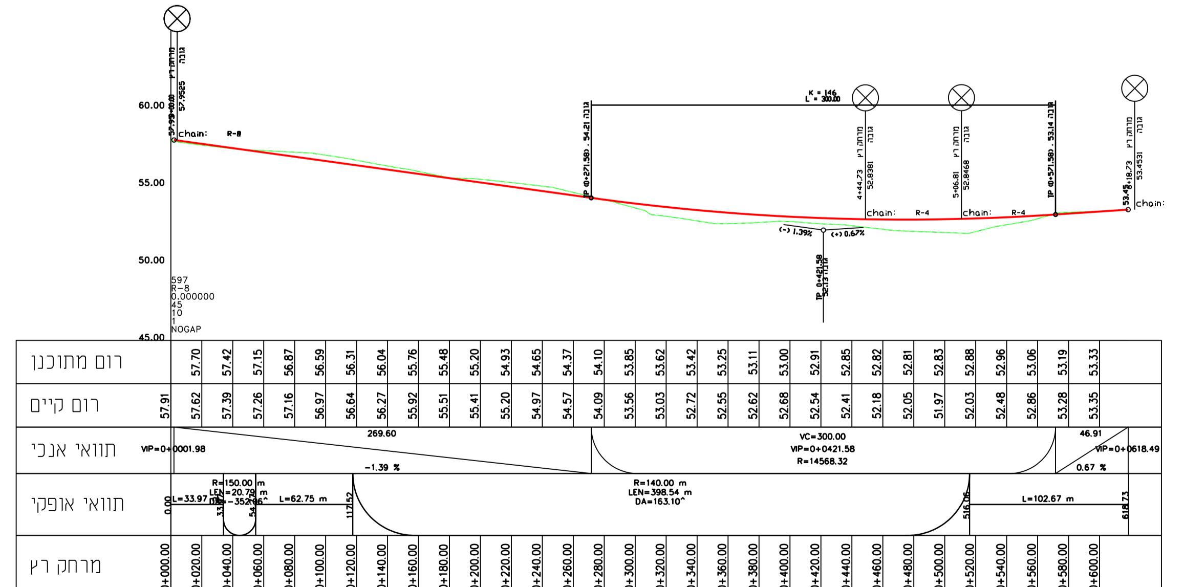
חתך לאורך דרך מסי' 08
