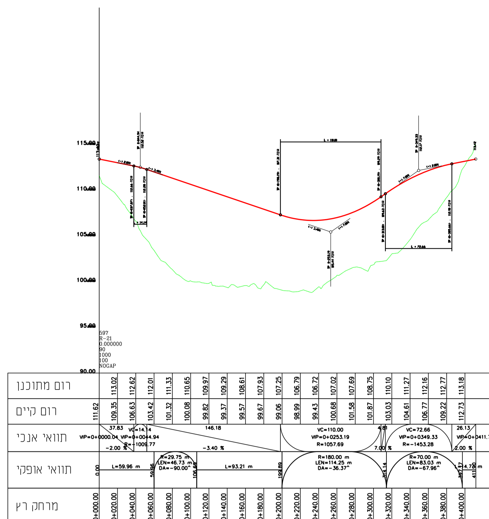
חתך לאורך דרך מסי' 21
