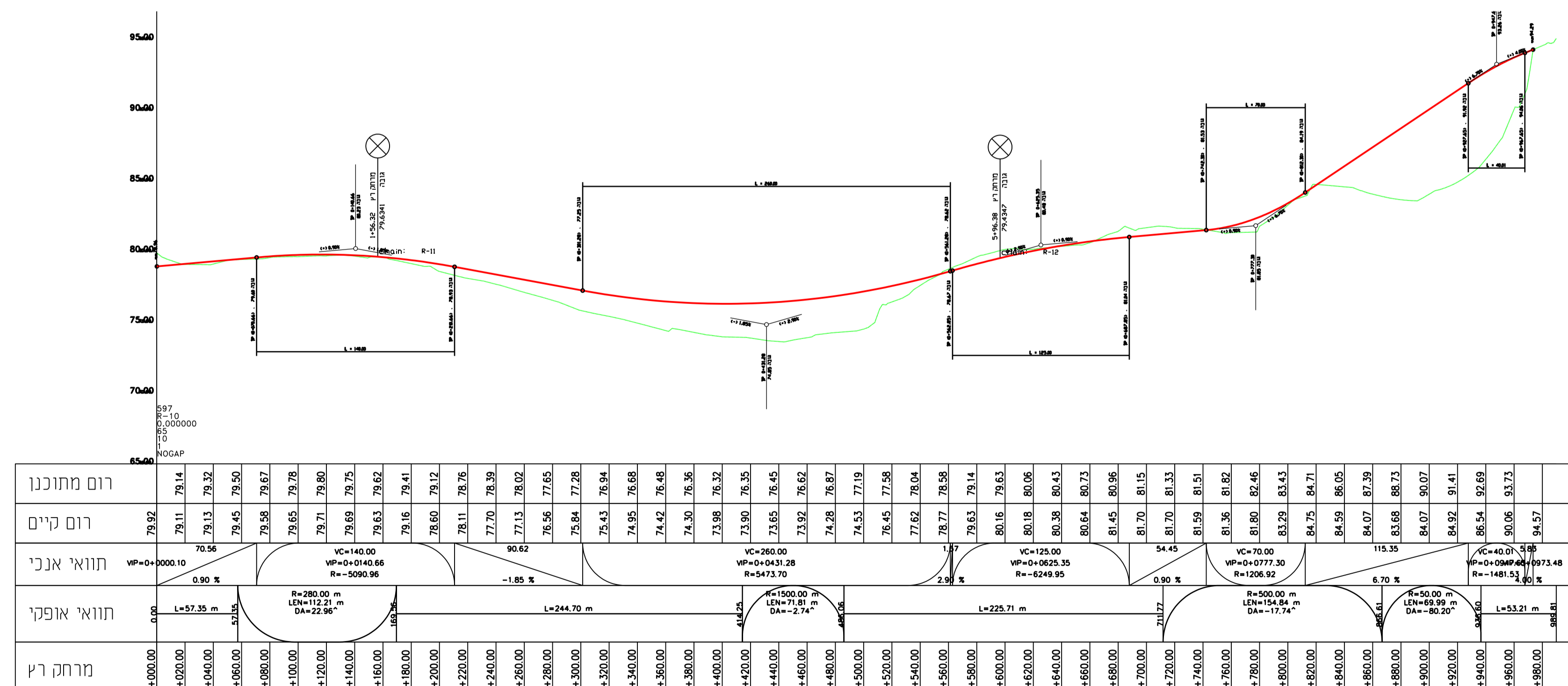
חתך לאורך דרך מסי' 10
