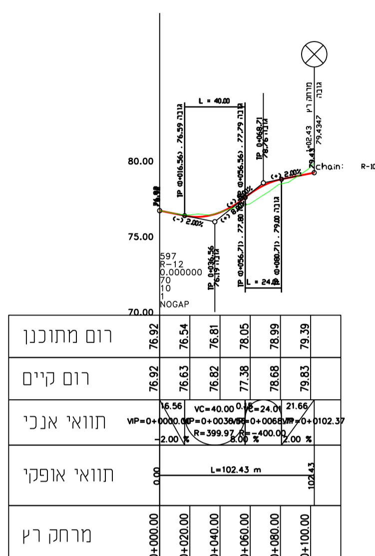
חתך לאורך דרך מסי' 12
