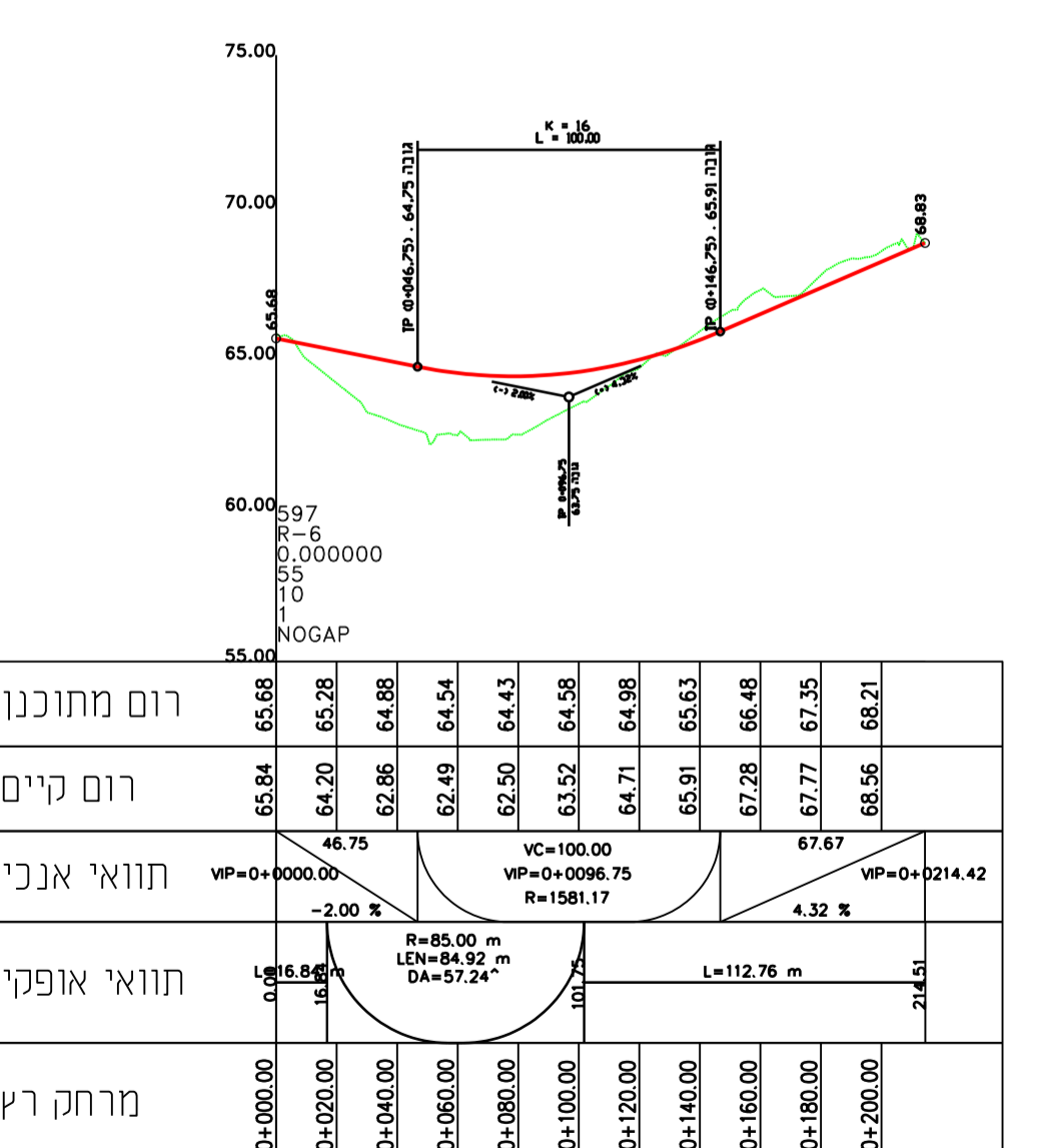
חתך לאורך דרך מסי' 06
