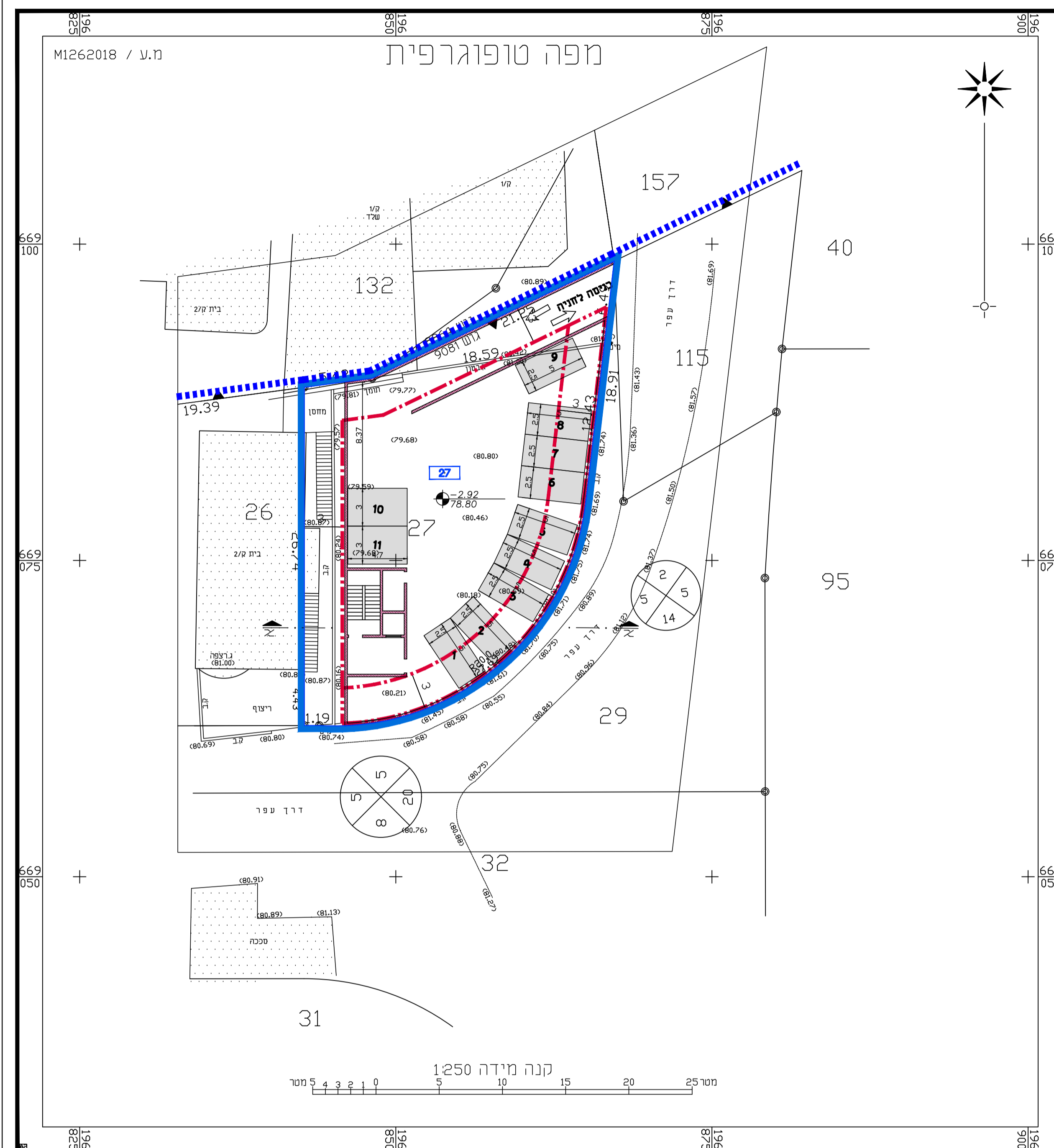
תכנית חניה קנ"מ 1: 250
