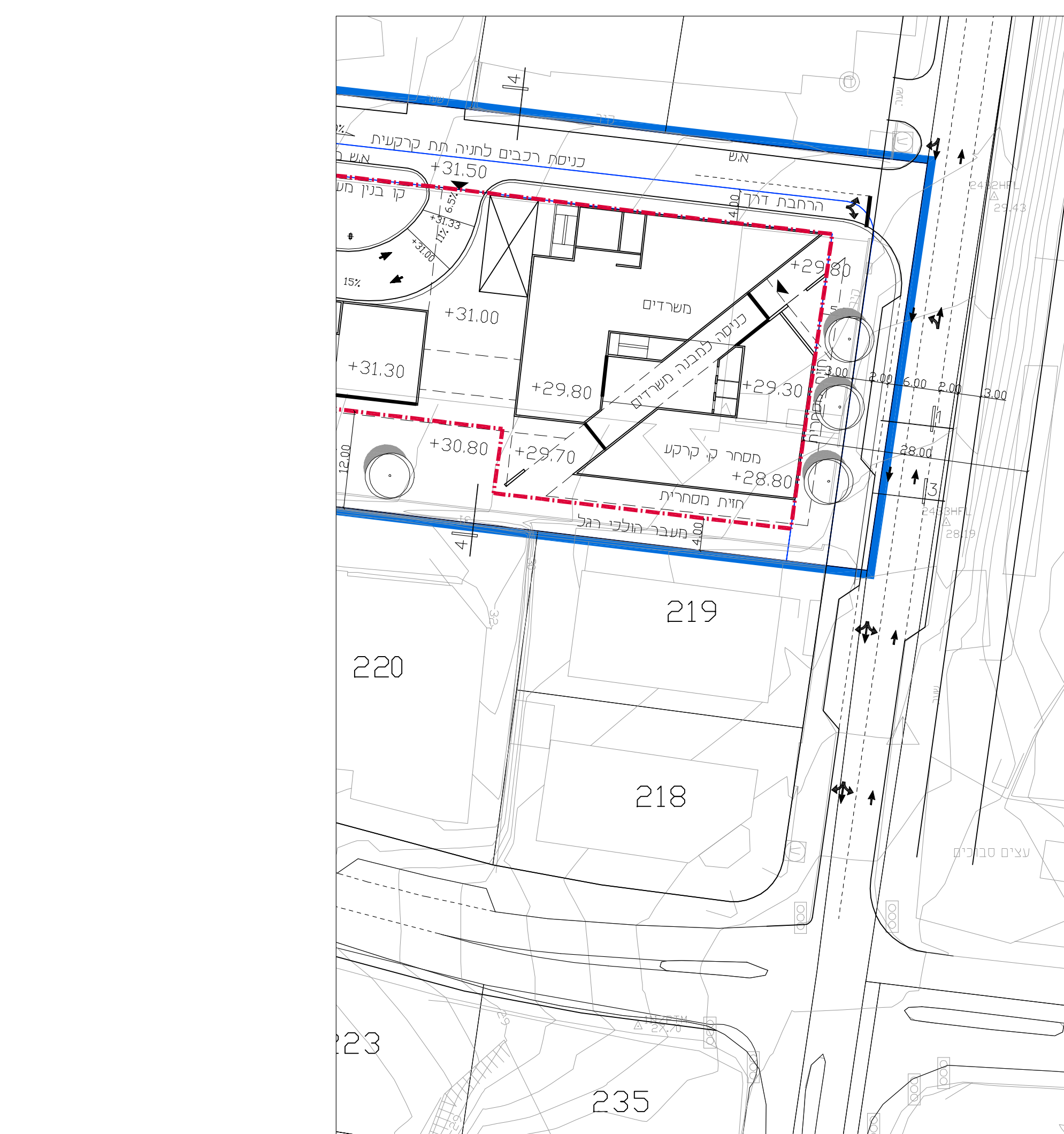
תכנית קומת הקרקע
