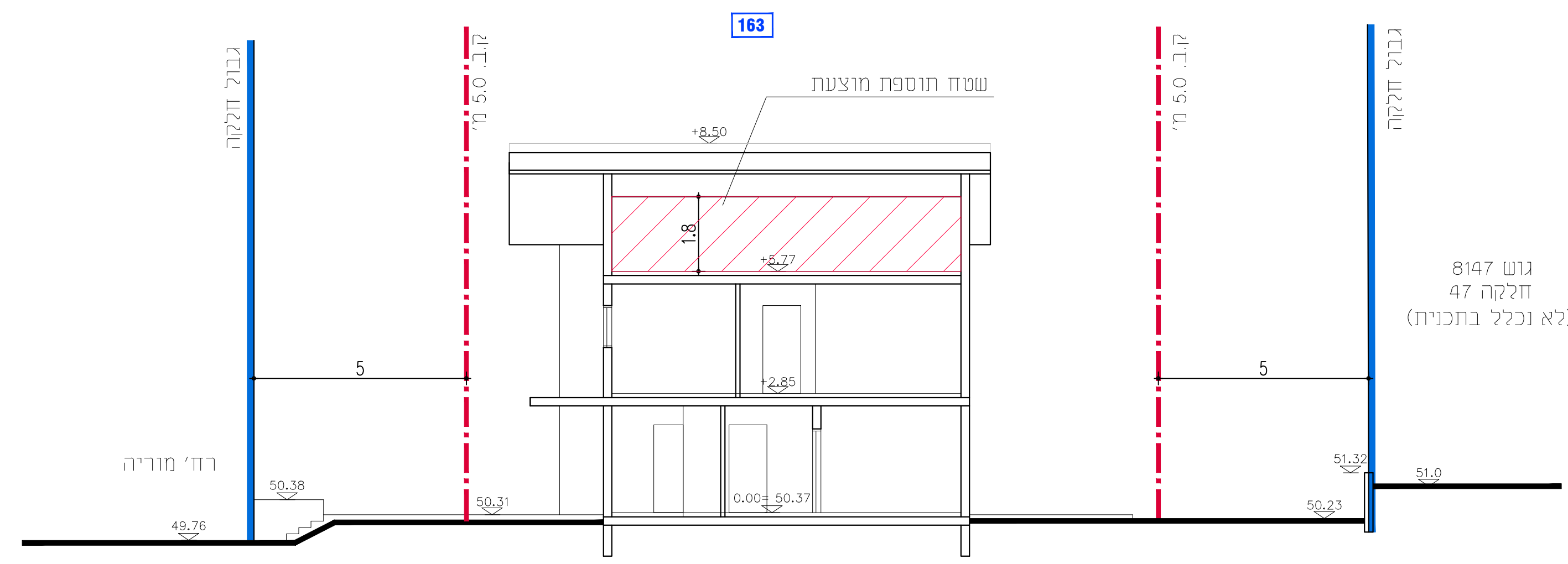
חתך ב-ב קנ"מ 1:100
