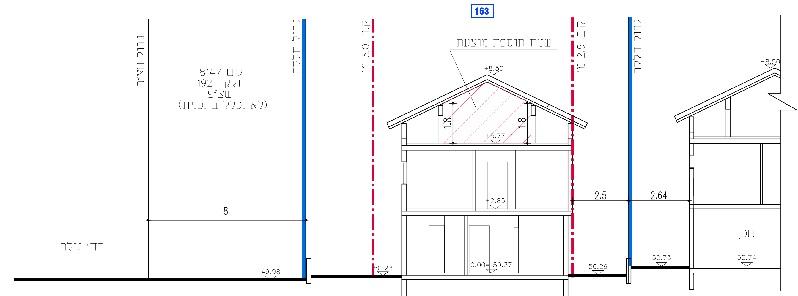
חתך א-א קנ"מ 1:100
