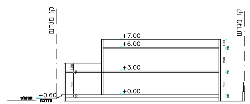
חזתן א א 1:250
