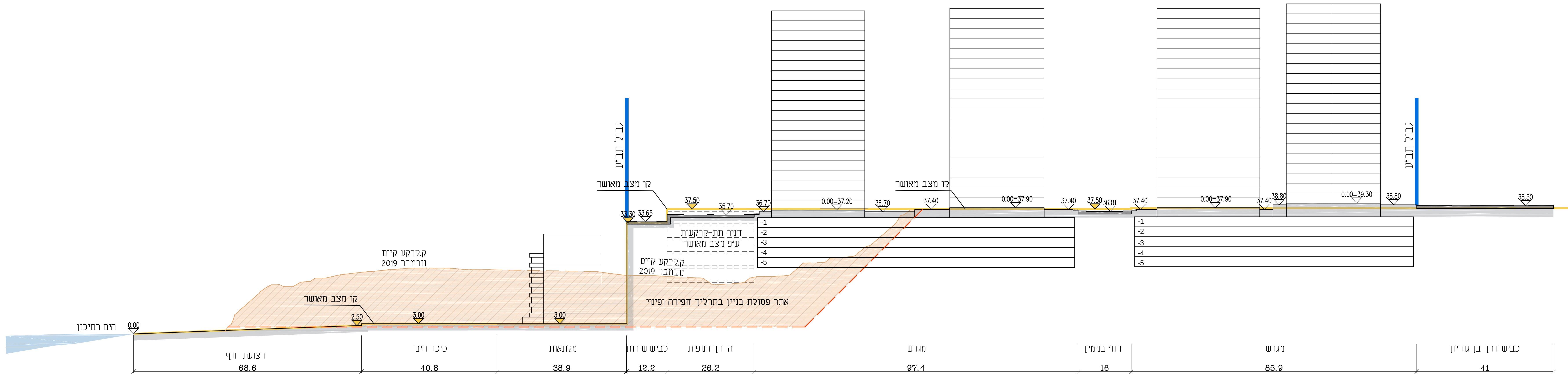
חתך א-א קנ"מ 1:500 מצב מוצע ומצב מאושר ביחס לאתר פסולת
