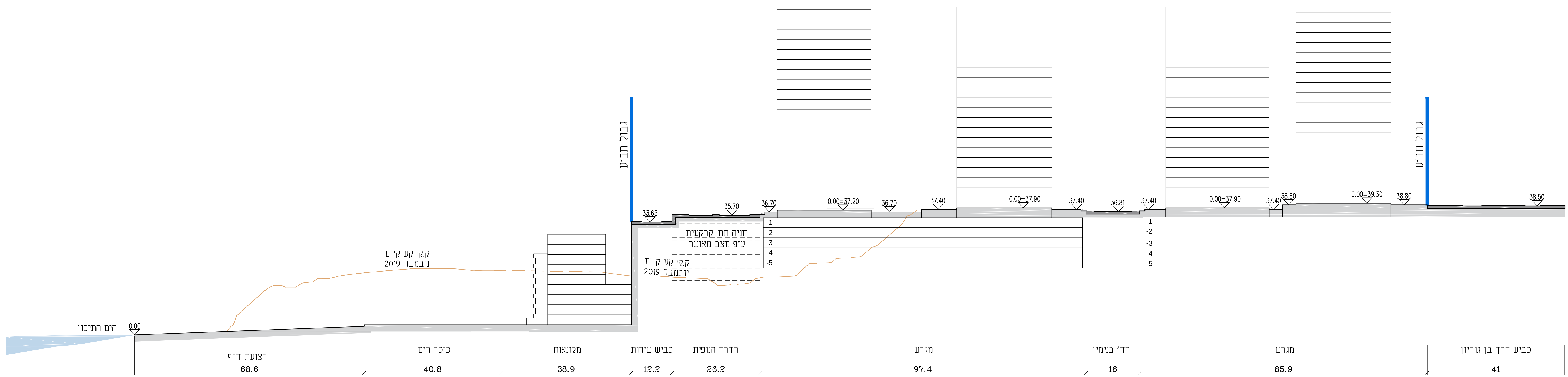
חתך א-א קנ"מ 1:500 מצב מוצע
