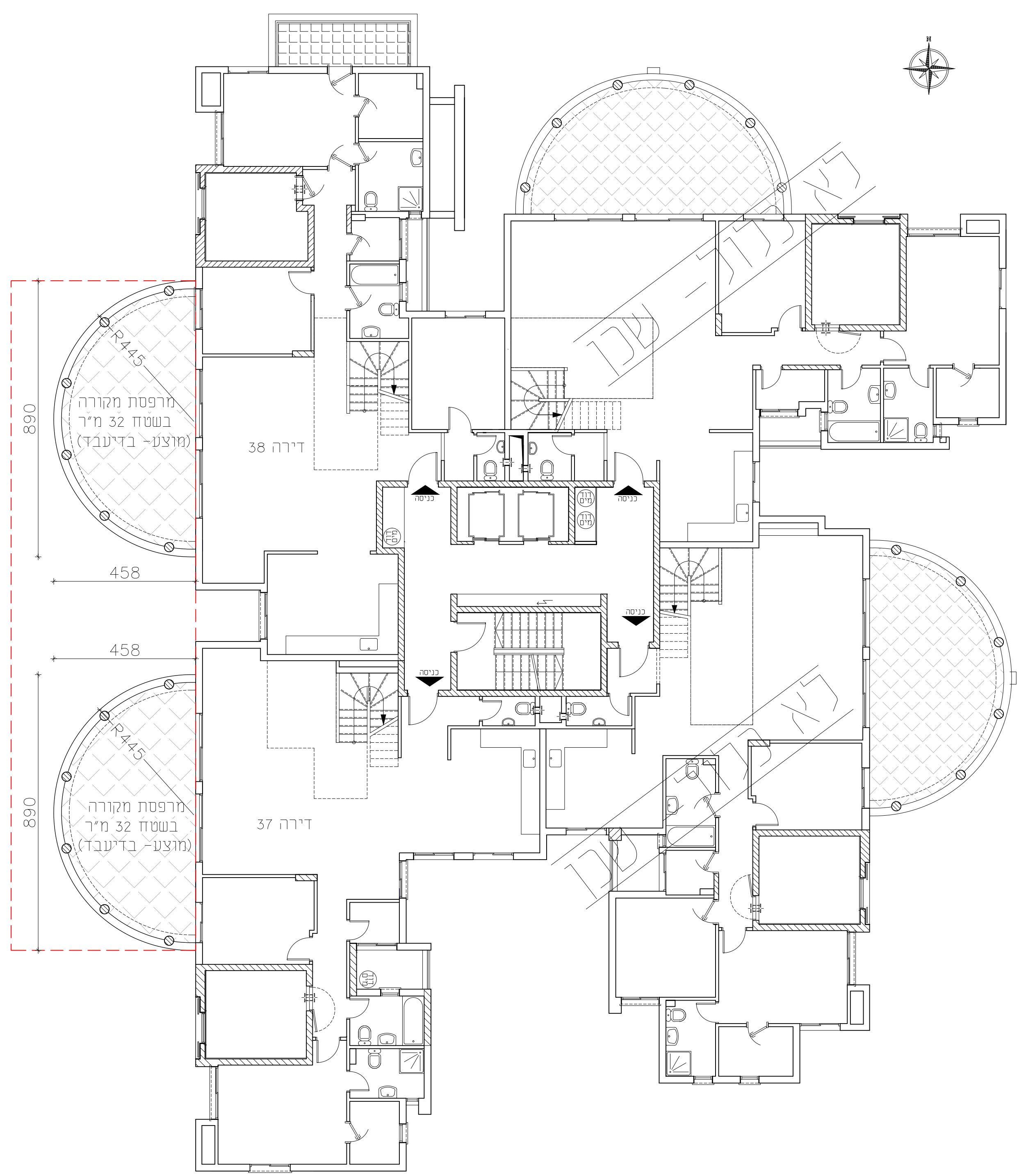
קומה תשיעית - מפלס +26.90
