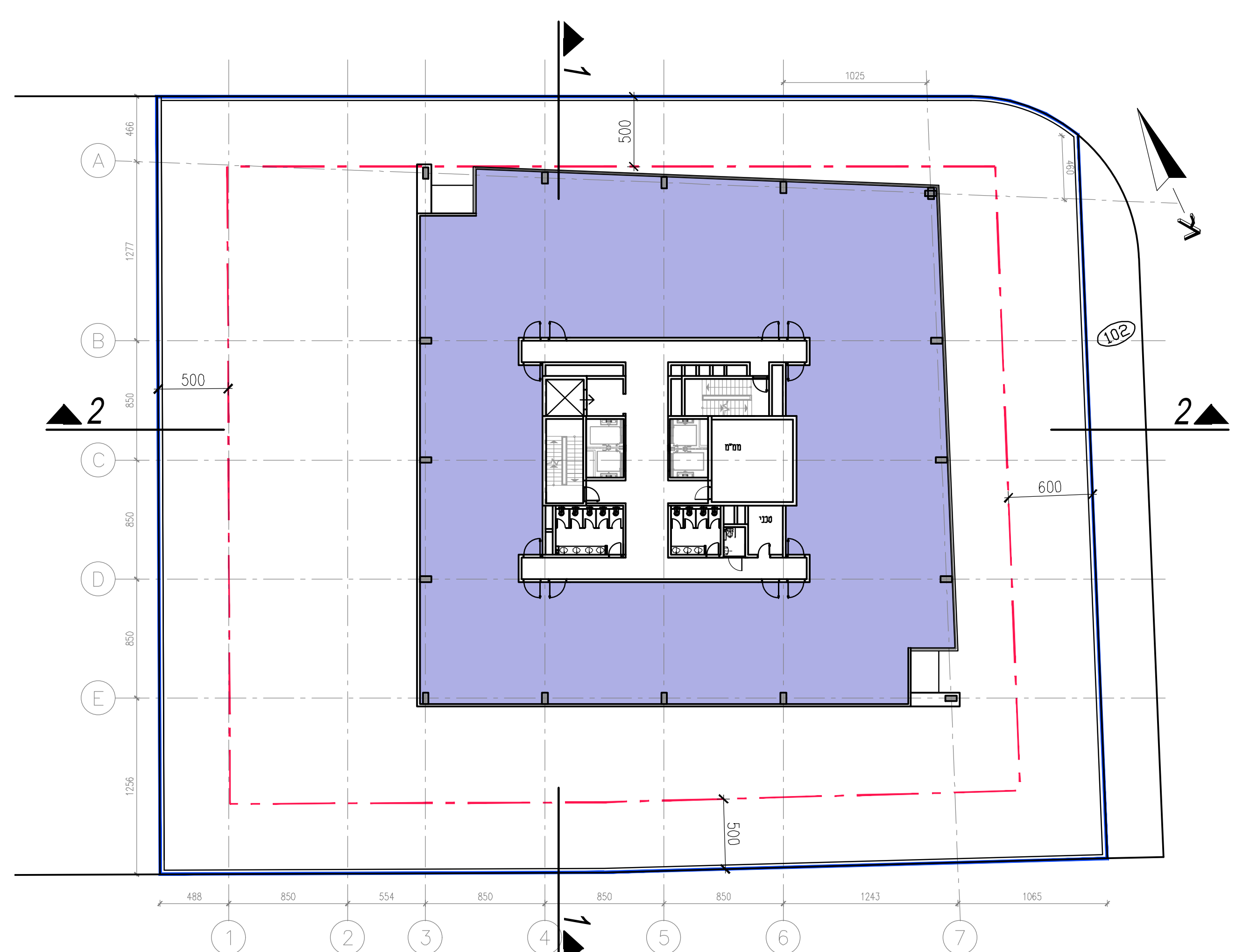
קומה טיפוסית
