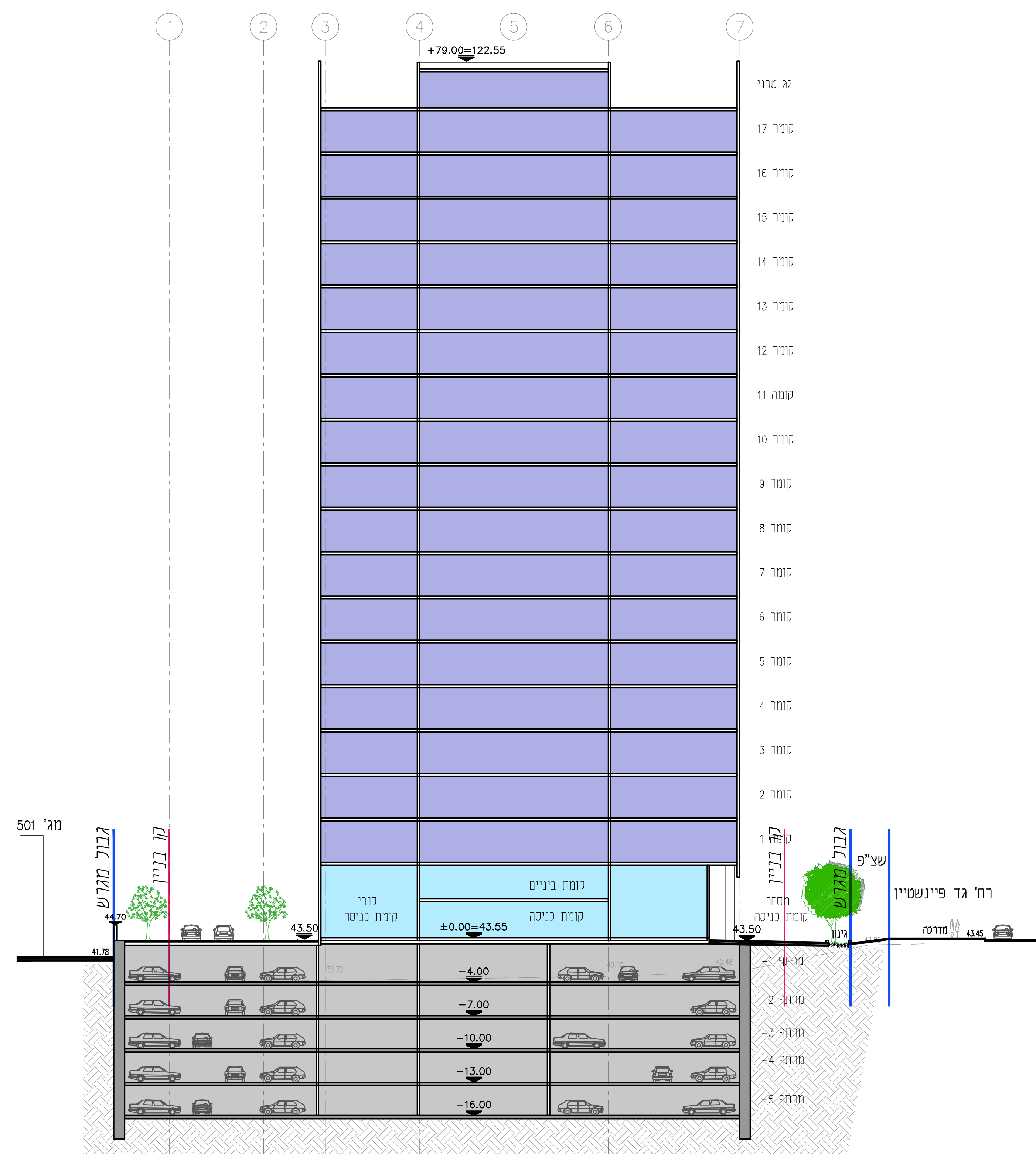
חתך עקרוני 2-2
