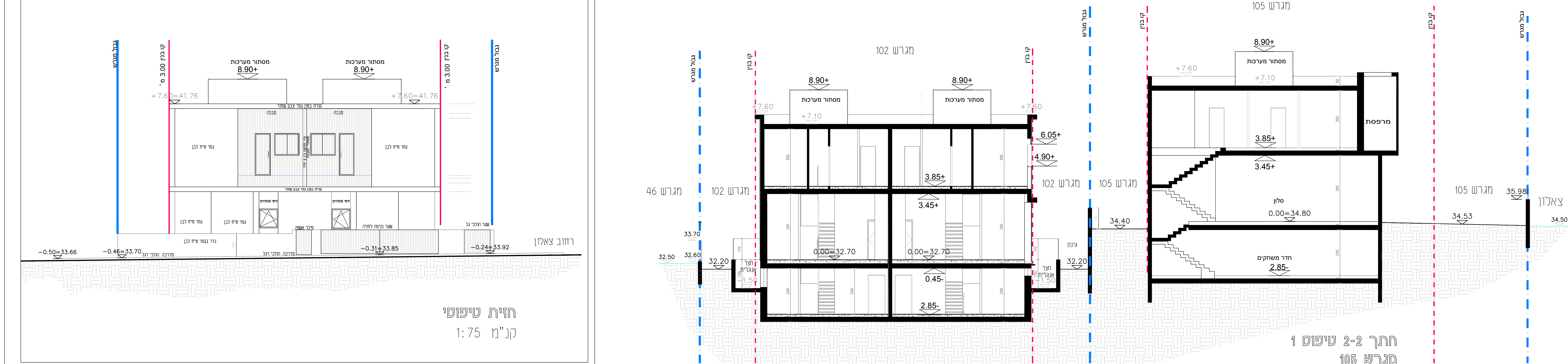
חתך 1-1 טיפוס 1
