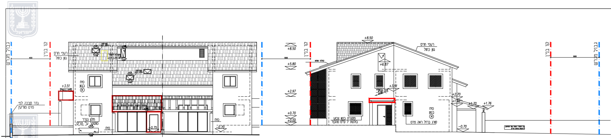
חזית אחורית 1:200
