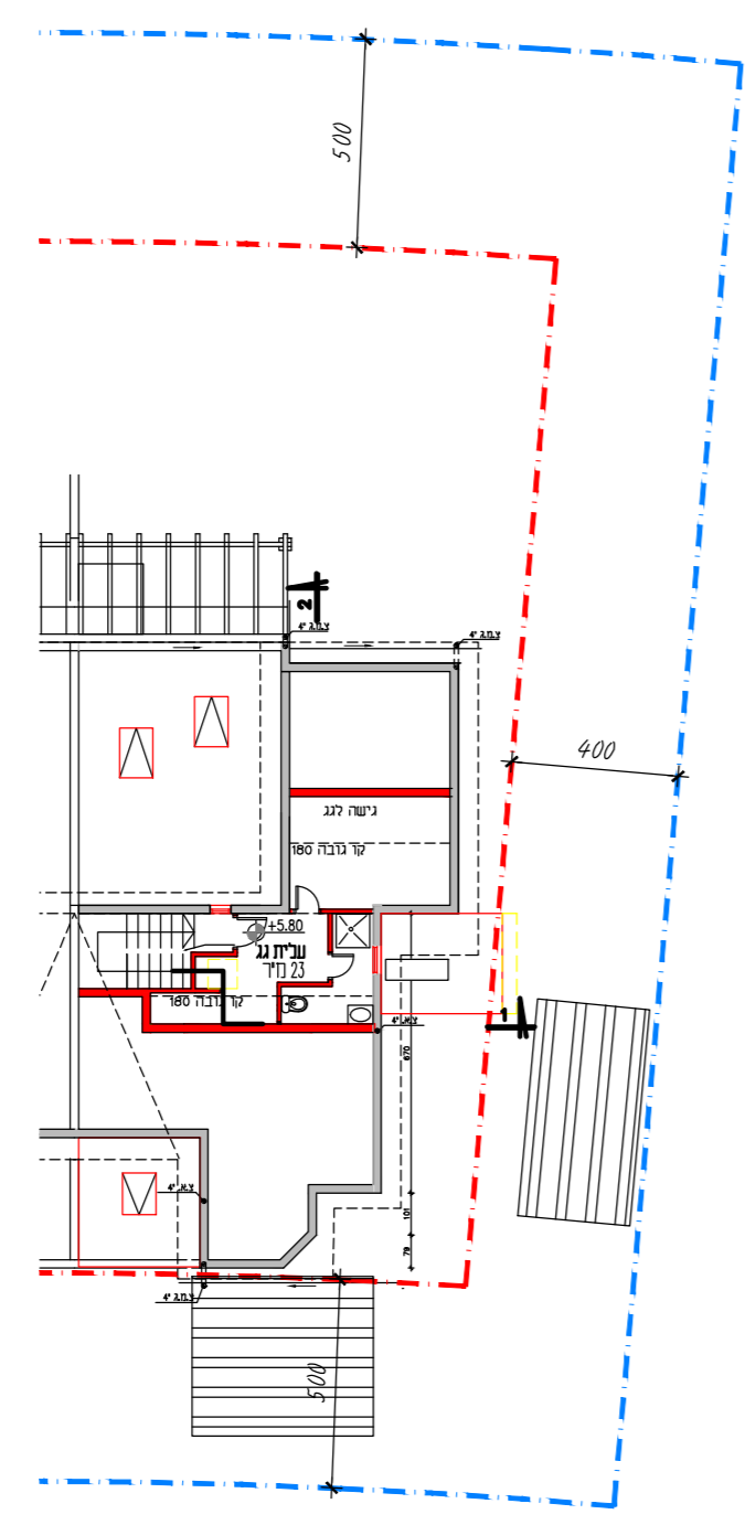
עלית גג 1:200
