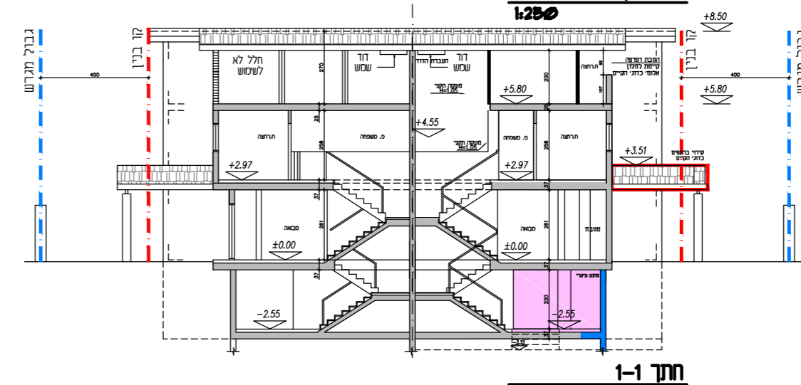
חתך 1-1 1:200
