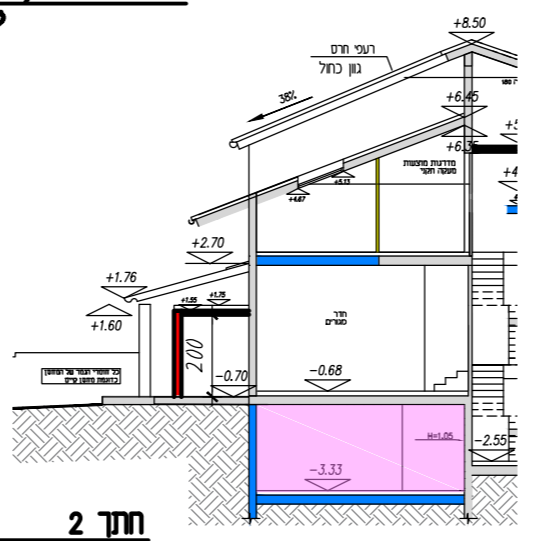
חתך 2 1:200
