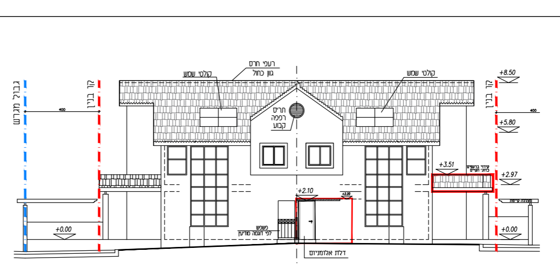
חזית קדמית 1:200
