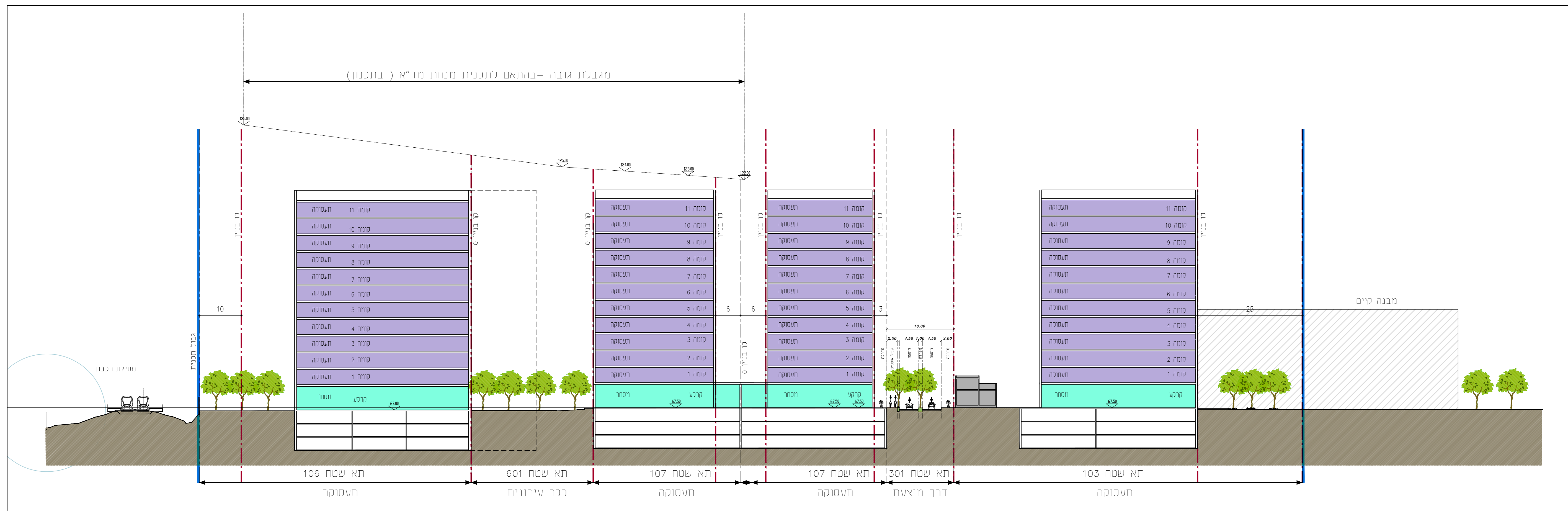
חתך א-א
