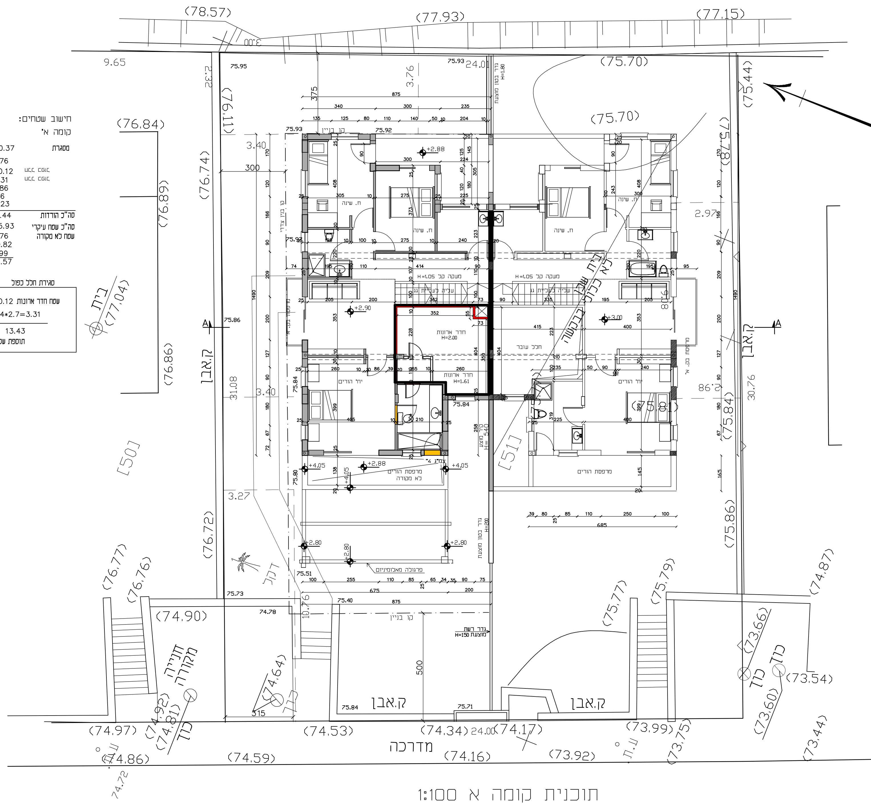
תוכנית קומה א 1:100
