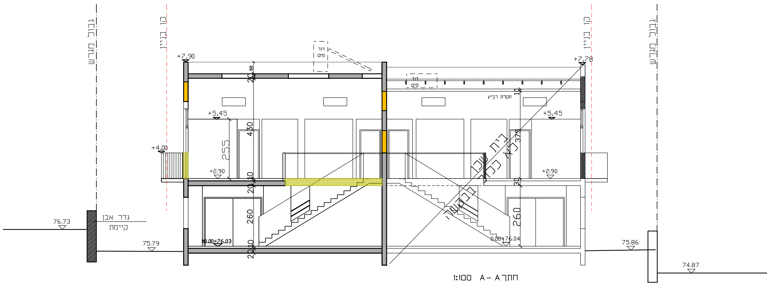
חיתוך A-A סכום
