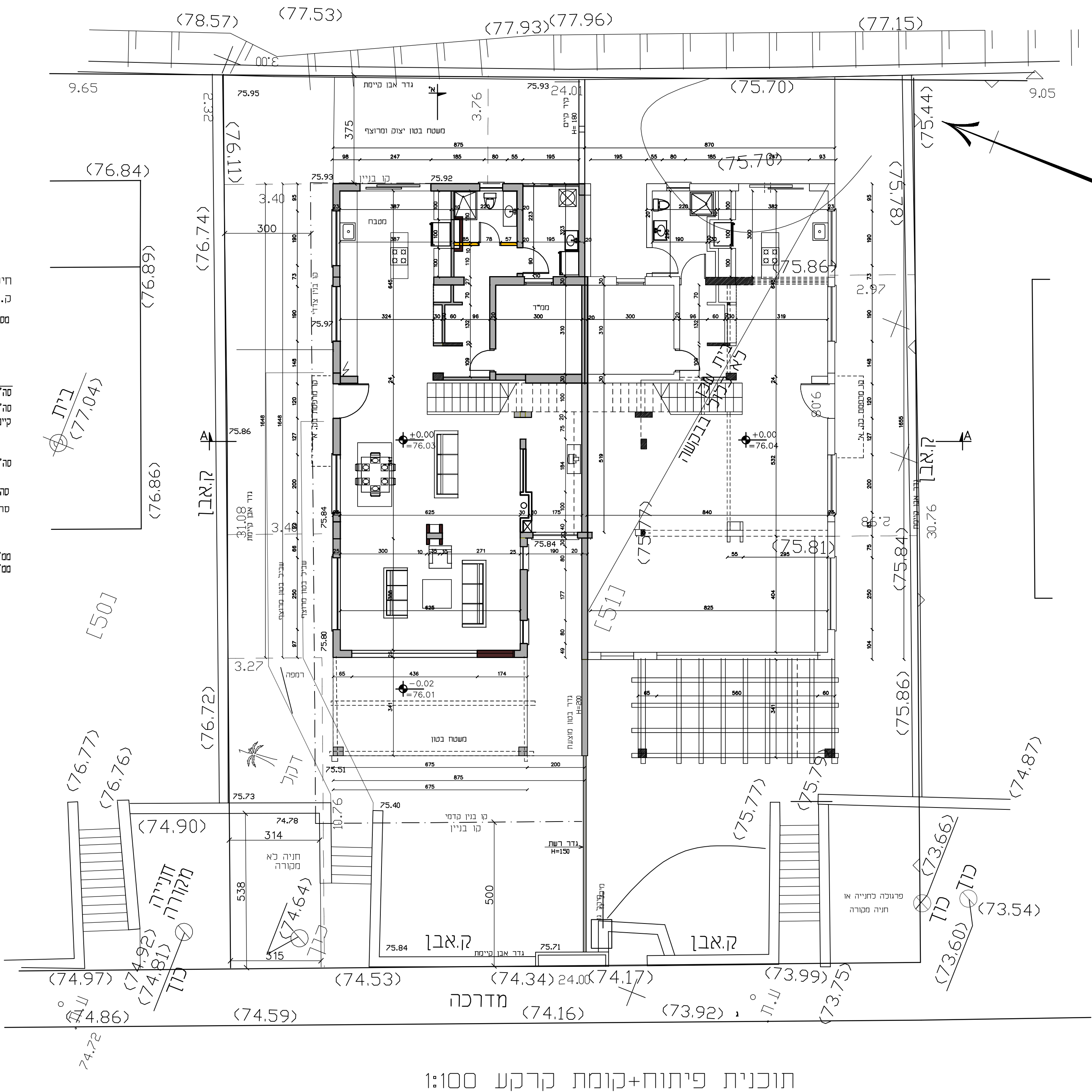
תוכנית פיתוח+קומת קרקע 1:100
