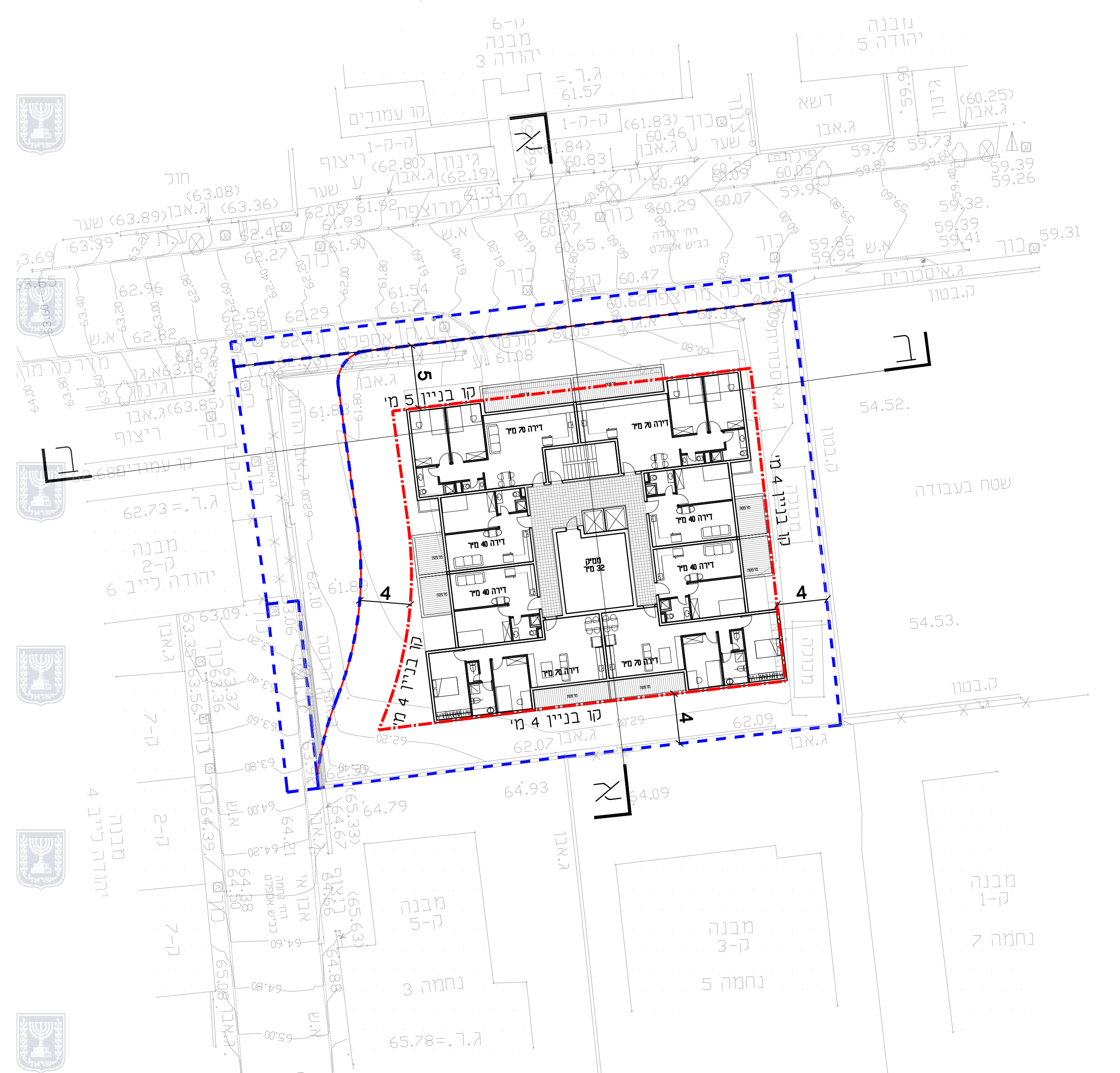
קומת טיפוסית מגורים קנ"מ 1:250
