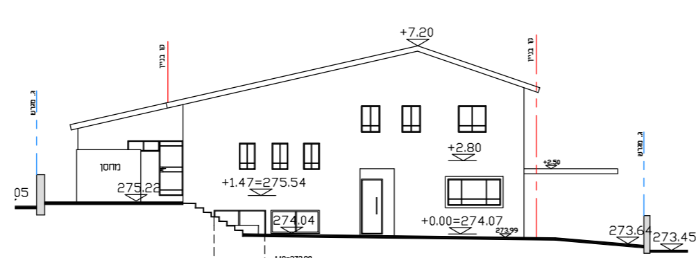
חזית צפונית 1:200
