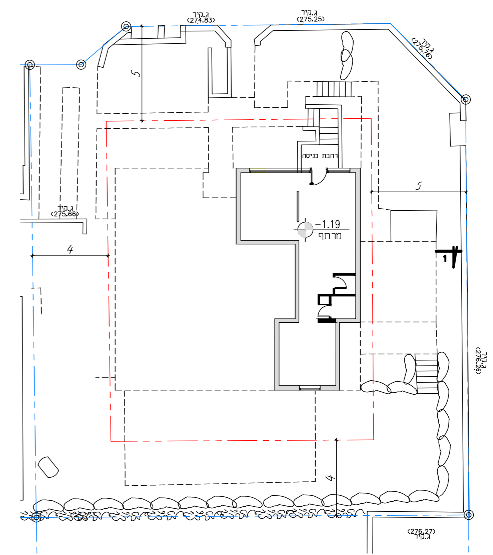
בוסת מרתף 1:200
