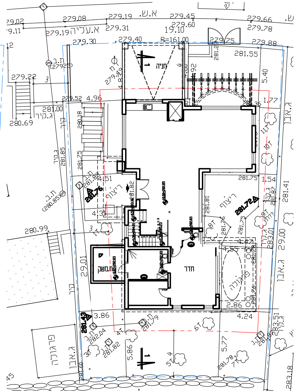
קומת קרקע 1:250
