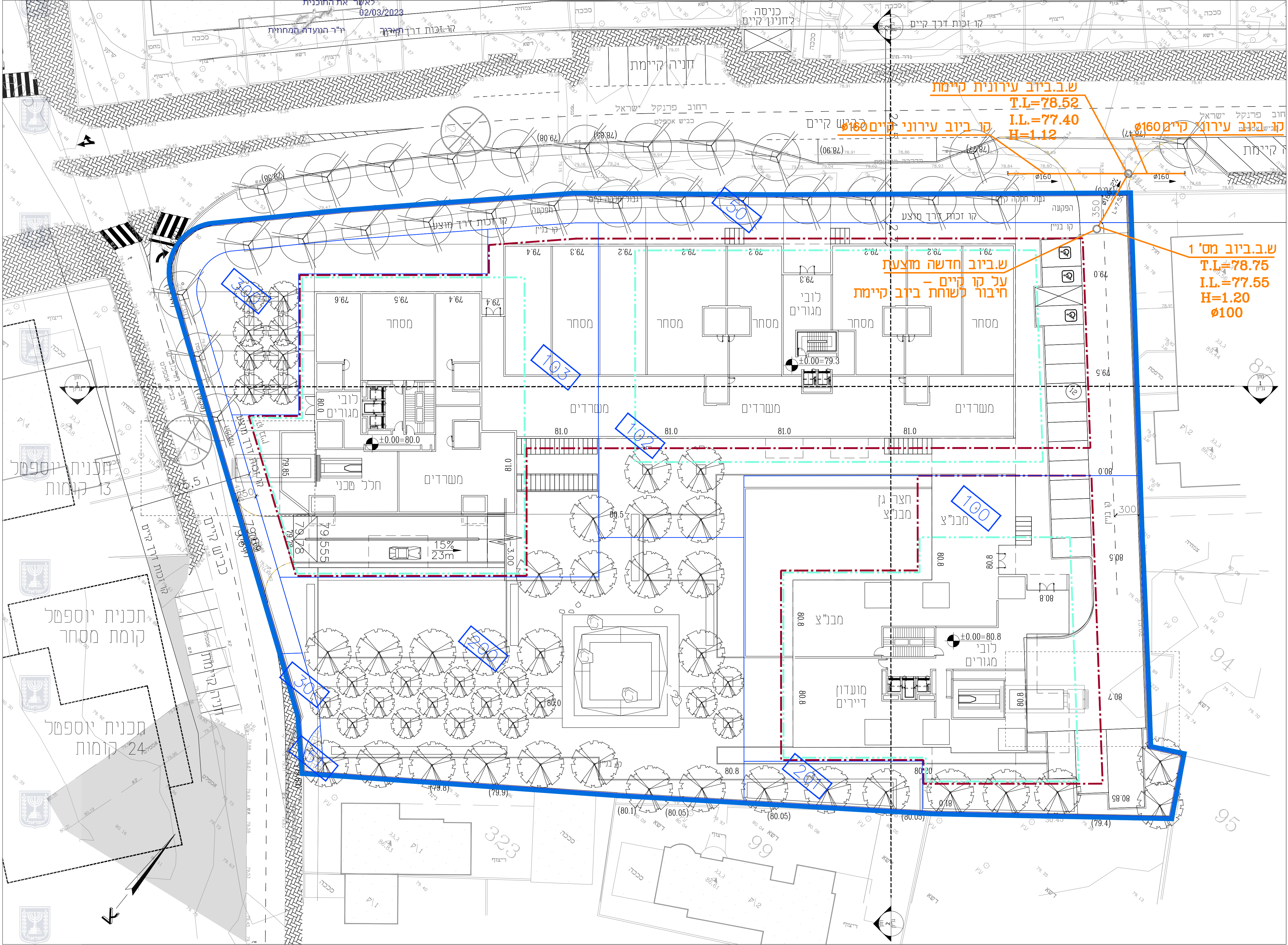
תכנית קומת קרקע 1:250
