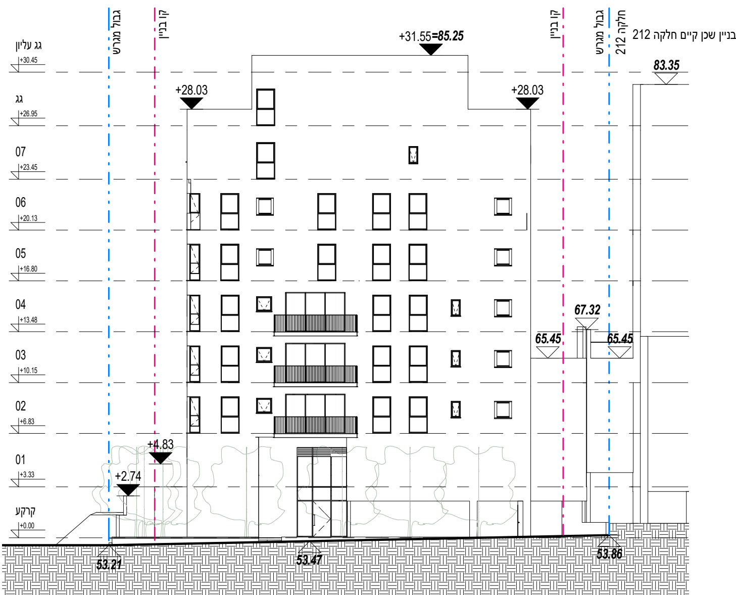
חזית צפונית
