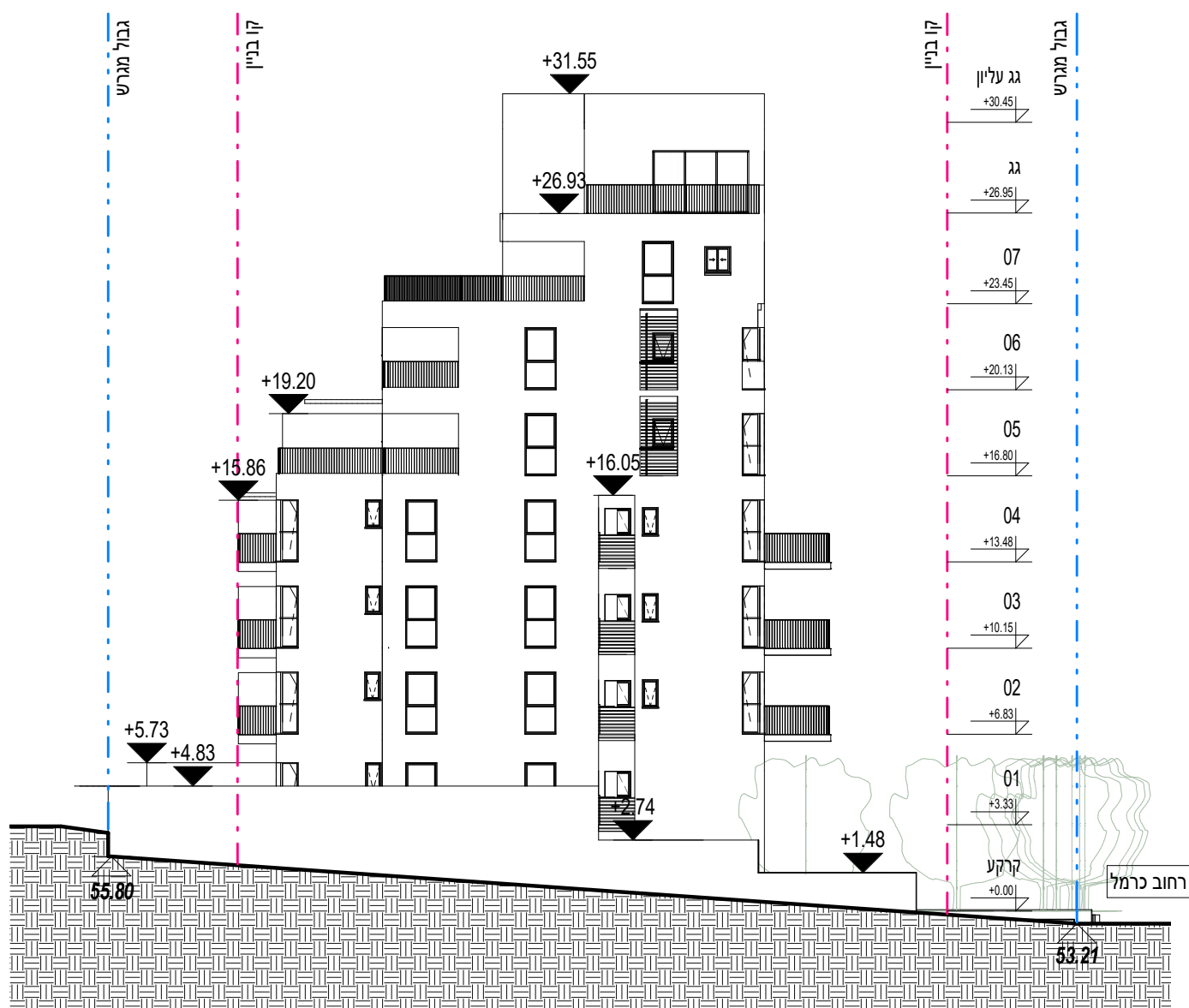
חזית מזרחית
