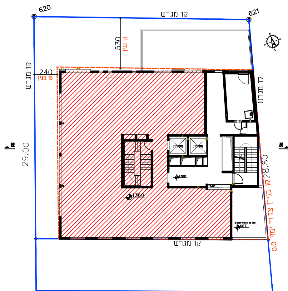
קומה ד ק.מ. 1:250
