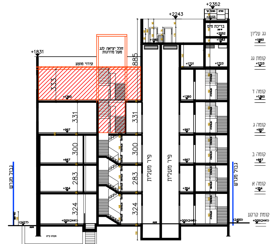
חתך א-א ק.מ. 1:250
