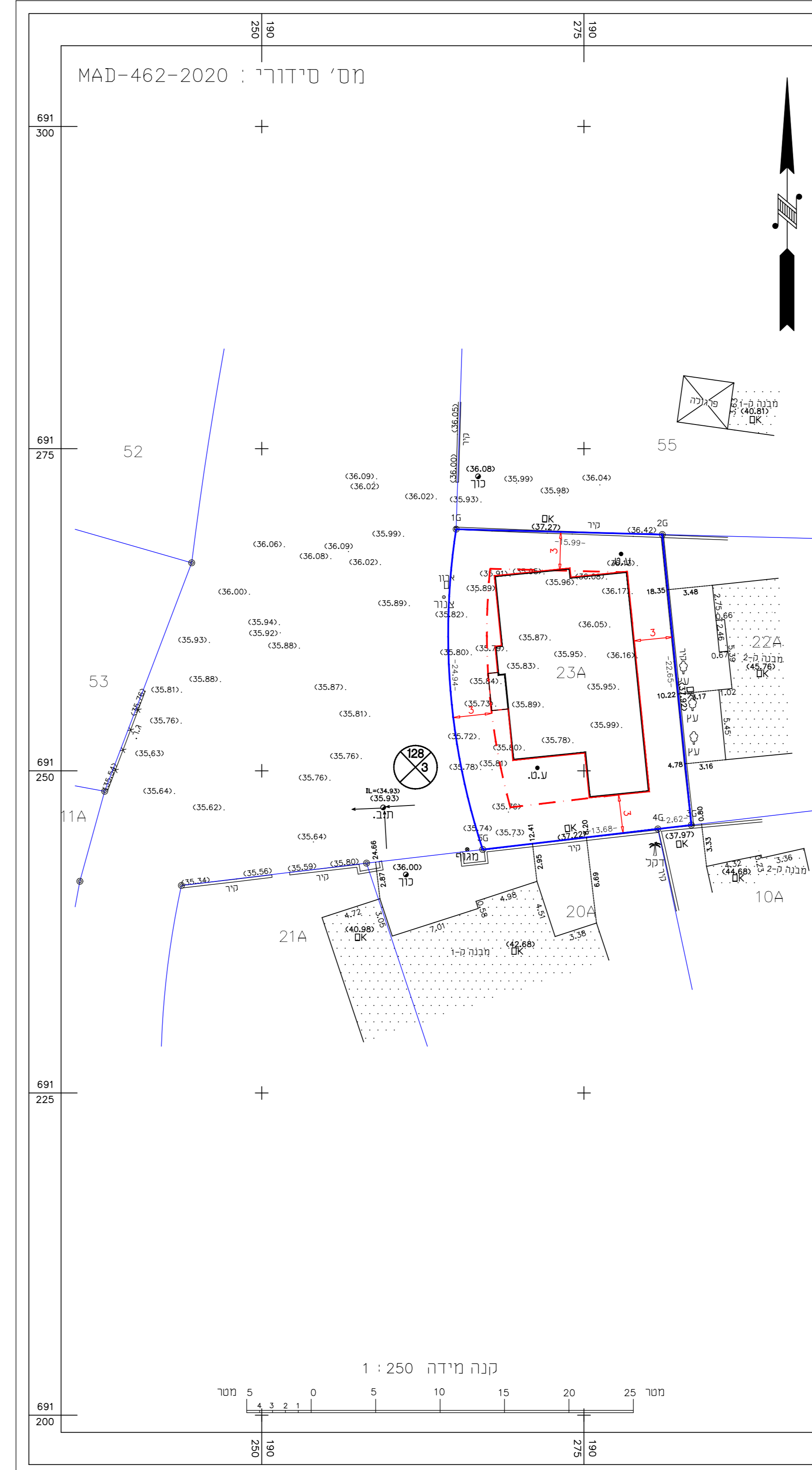
תכנית העמדה קנ"מ 1:250
