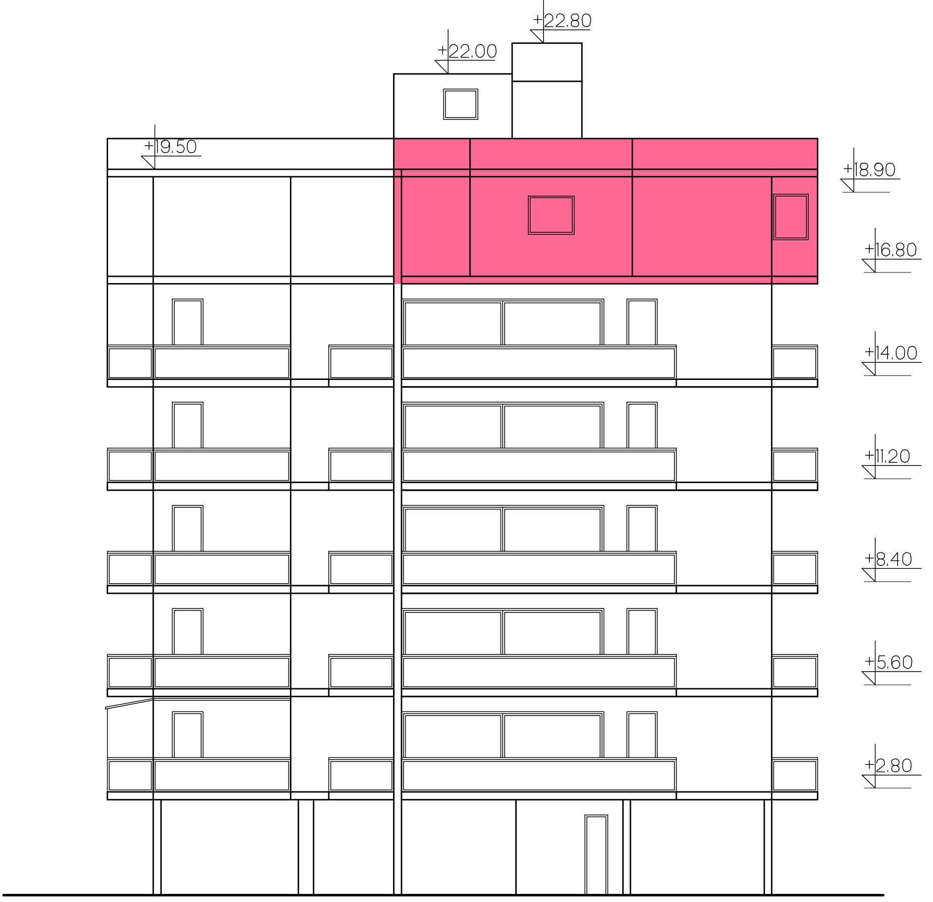
חזית מערבית 1:250
