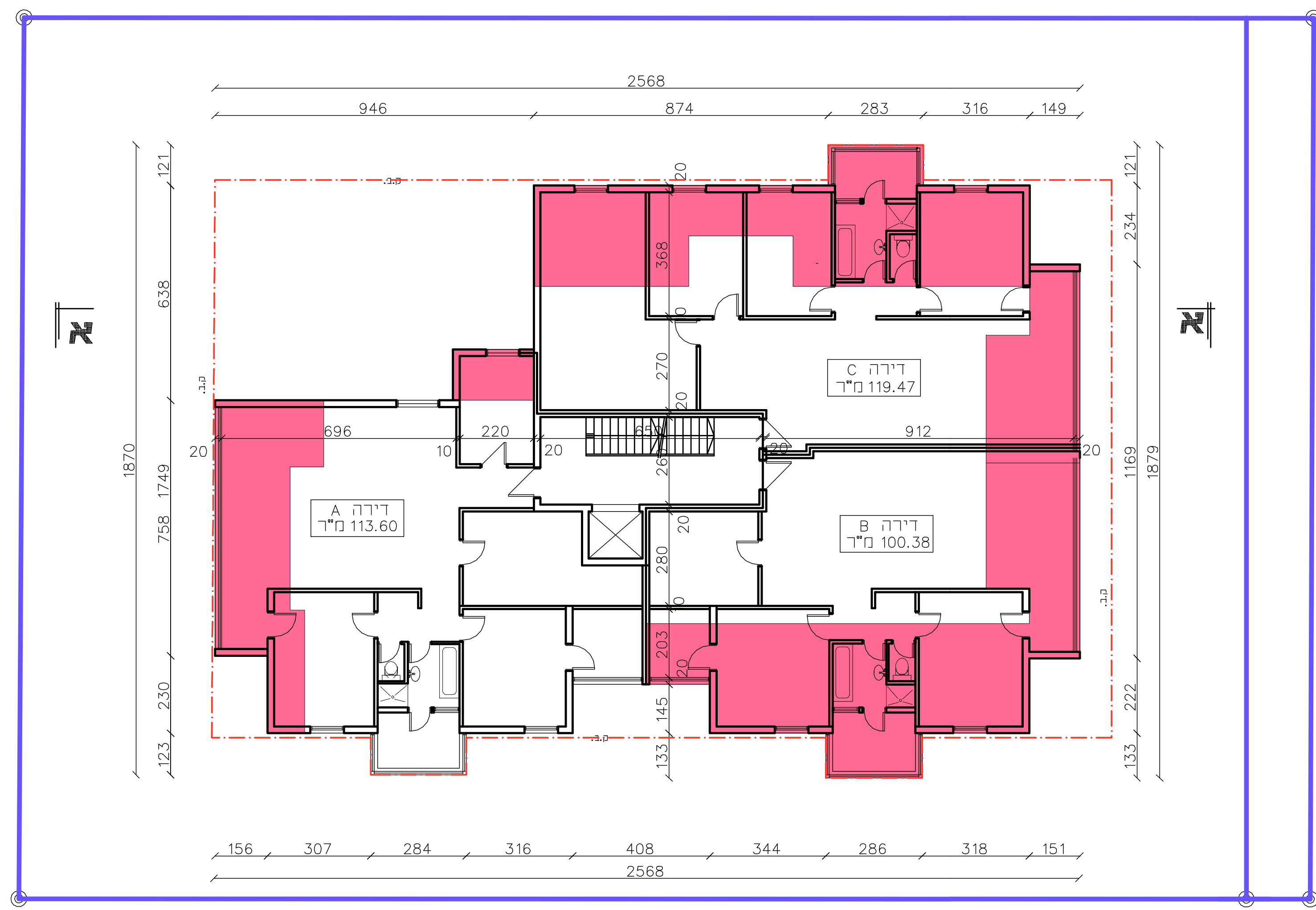
קומה ו' 1:100
