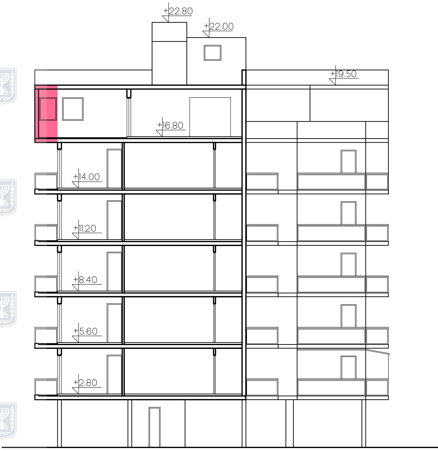
חתך א'-א' 1:250
