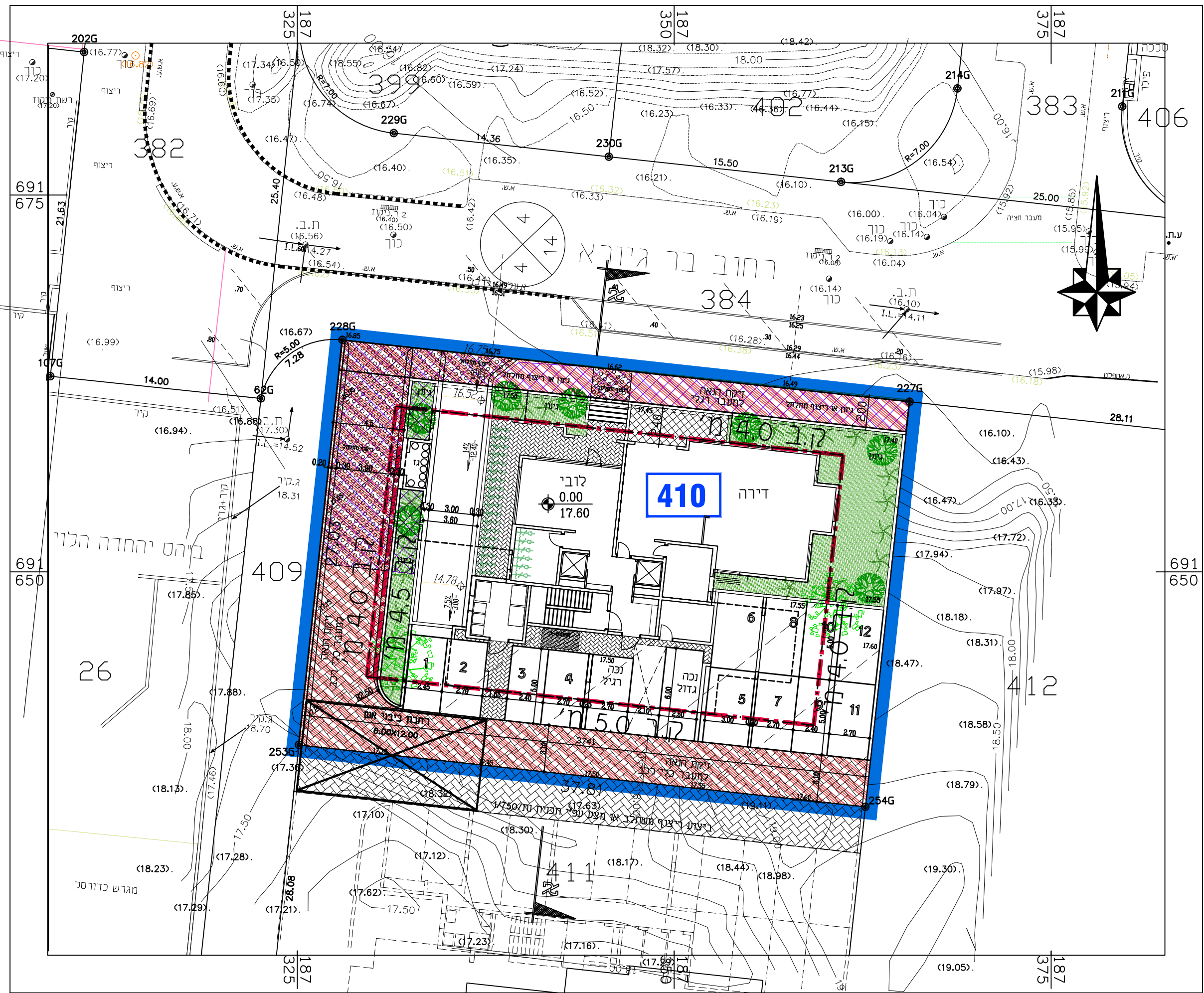
קומת קרקע קנ"מ 1:250
