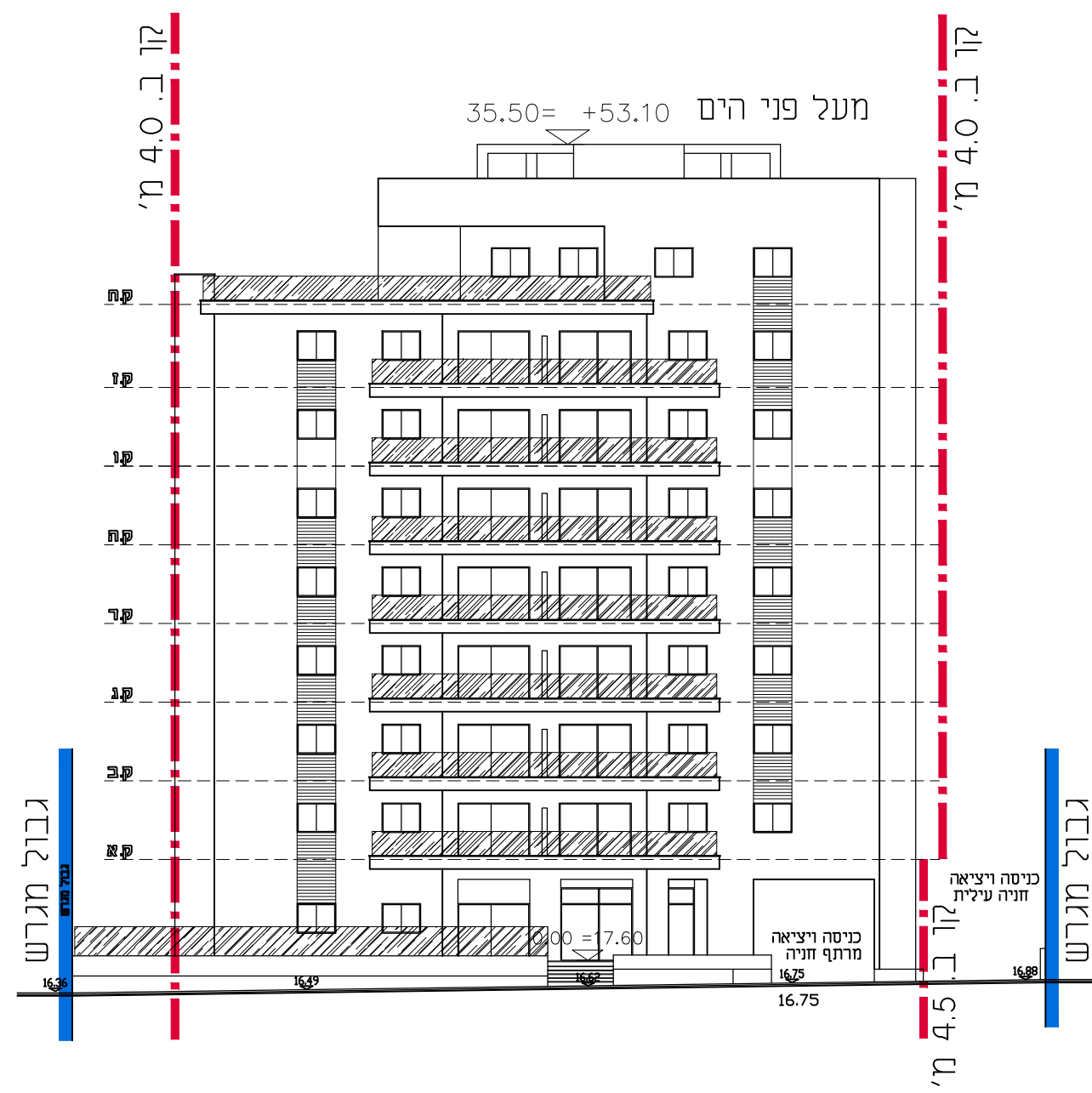
חזית ב-ב' קנ"מ 1:250
