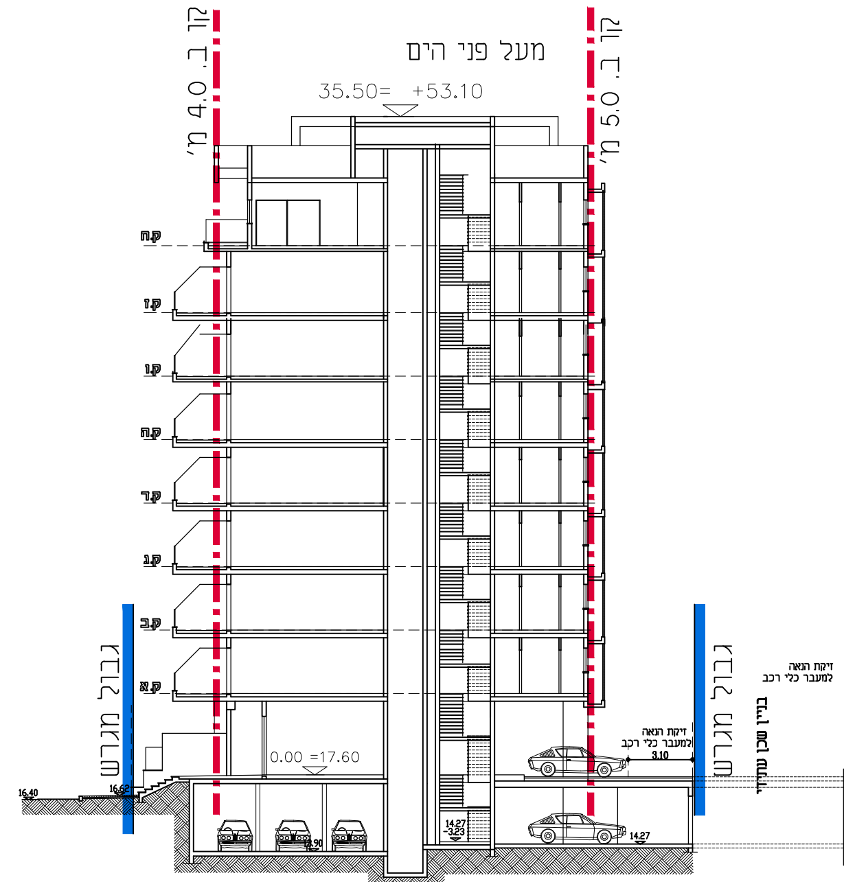
חזית א-א' קנ"מ 1:250
