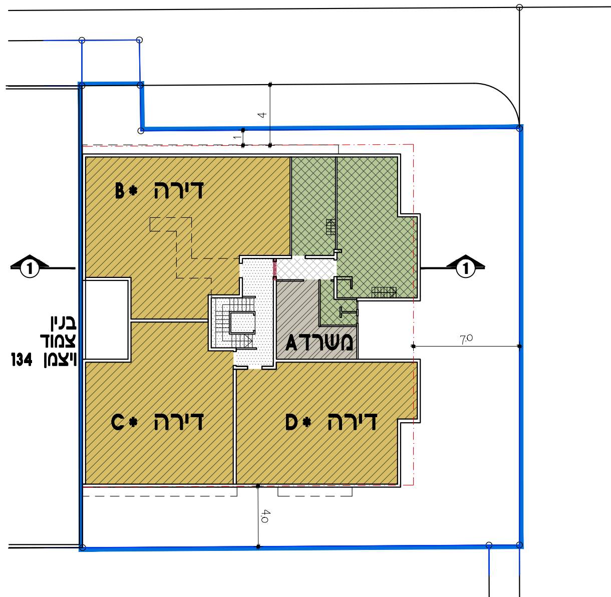
תכנית קומת גלריה 1:250
