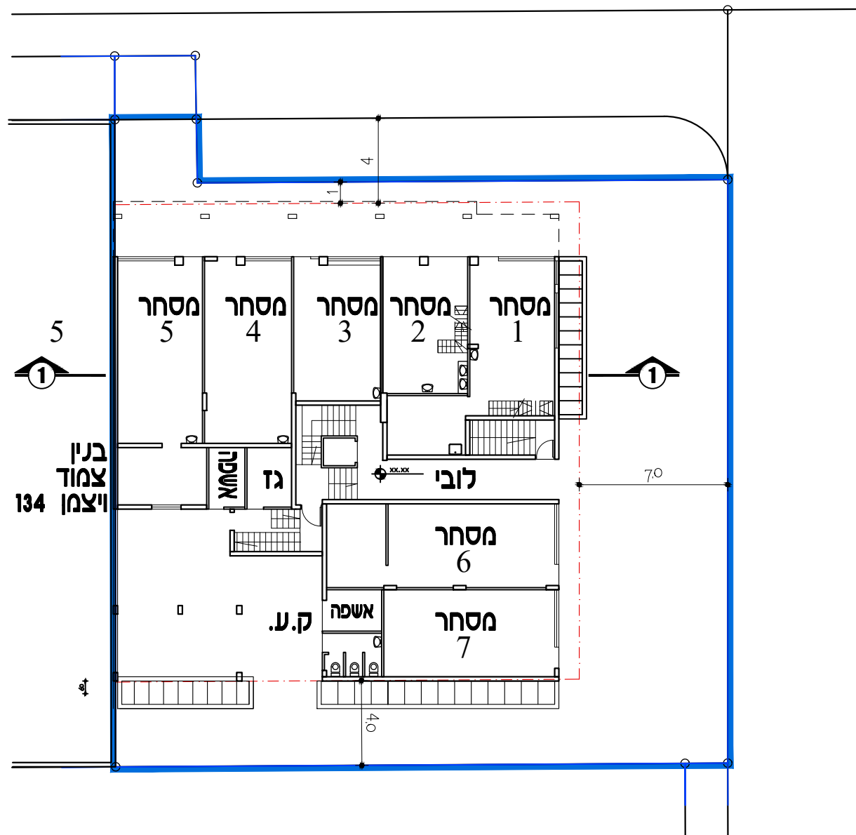
תכנית קומת קרקע מסחר 1:250
