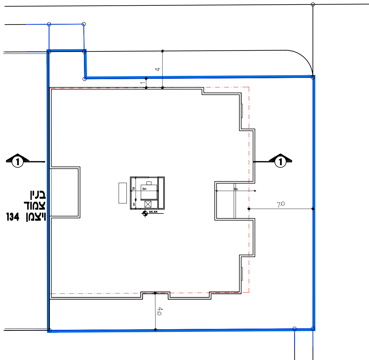
תכנית קומת גג 1:250
