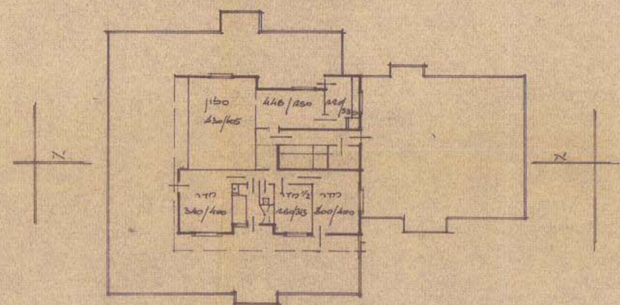
קטע קריס X Z ז 1:250 ק.מ.
