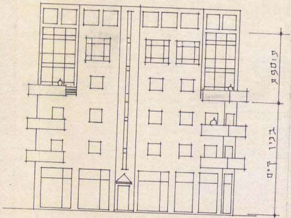
חזית דרומית ק.מ. 1:250
