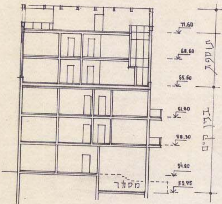
חתך א-א ק.מ. 1:250
