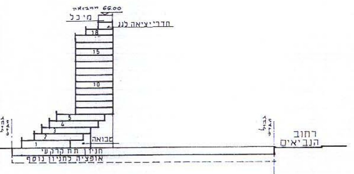
חתך עקרוני במגרשים 2-2-2-2 בתים בני 18 קומות
