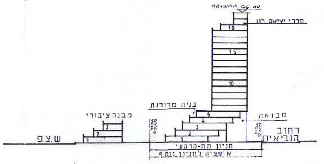
חתך עקרוני במגרש מ-4 בנין בן 19 קומות
